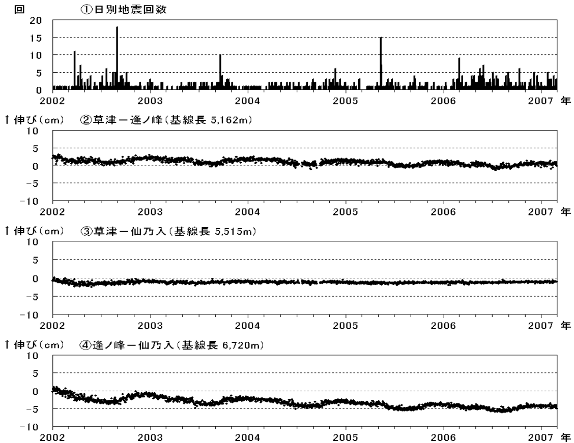
図 3 草津白根山 最近の火山活動の推移（2002 年 1 月～2007 年 2 月）
