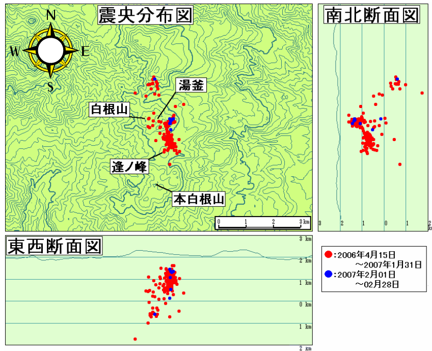
図 2※ 草津白根山 火山性地震の震源分布（2006 年 4 月 15 日～2007 年 2 月 28 日）
