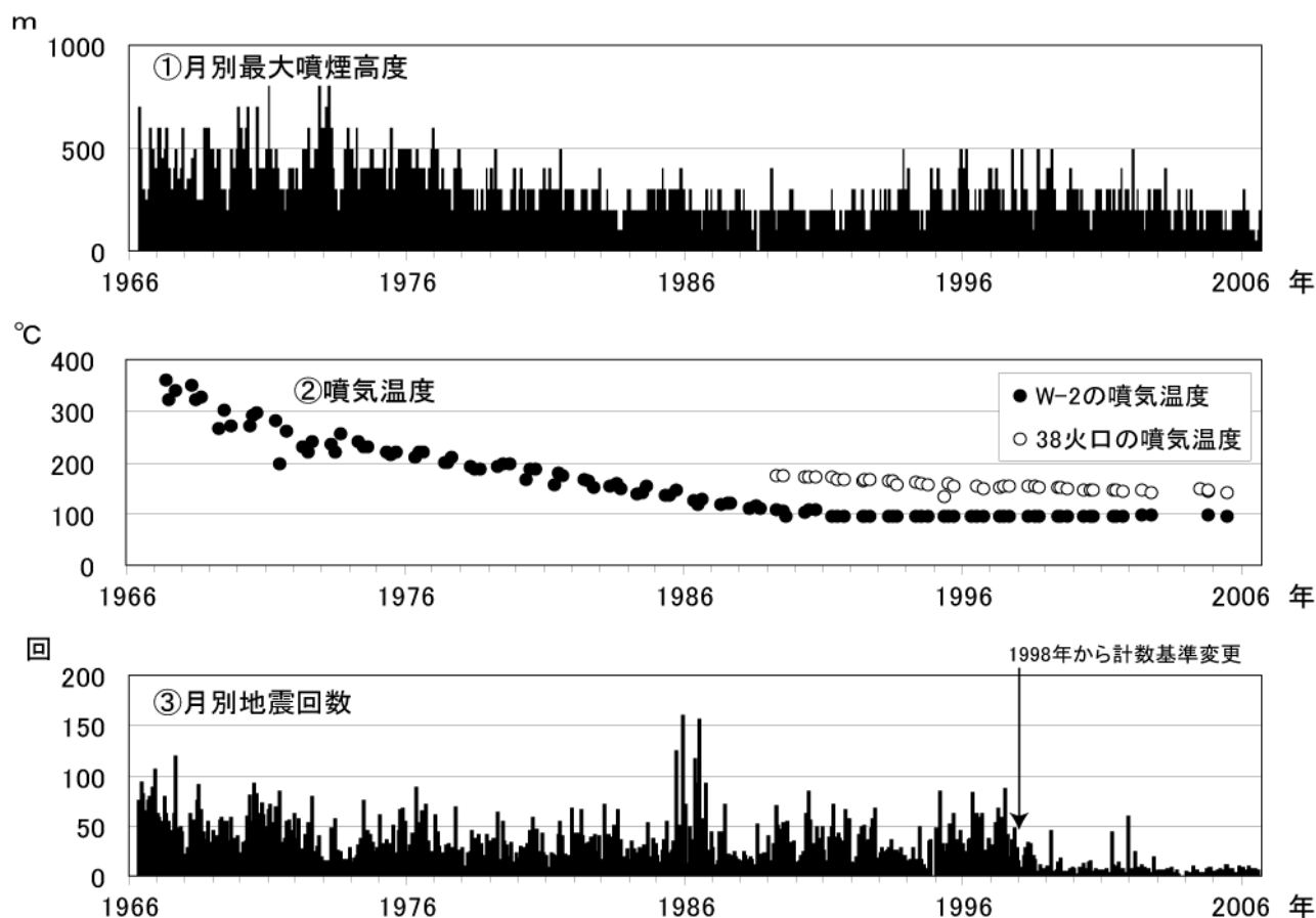
図 1 那須岳 最近の火山活動の推移（1966 年 1 月～2006 年 9 月）
