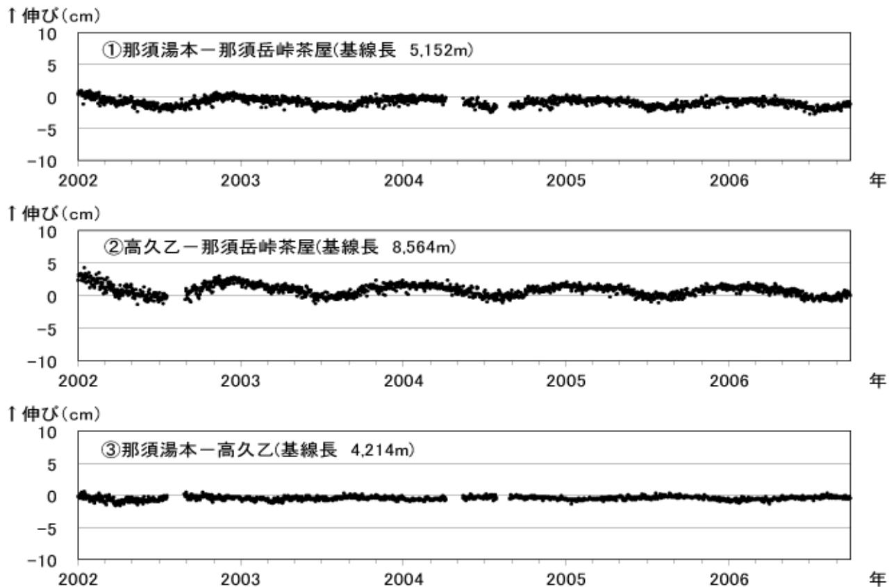
図3 那須岳 G P S 連続観測による基線長変化（2002年1月～2006年9月）
