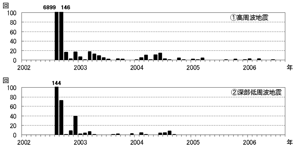
図 1 八丈島 月別地震回数（2002 年 8 月 13 日～2006 年 8 月 31 日）
