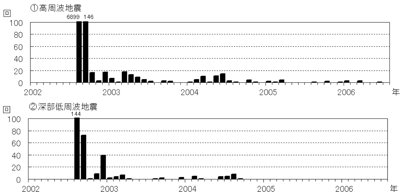
図 1※ 八丈島 月別地震回数（2002 年 8 月 13 日～2006 年 7 月 31 日）
