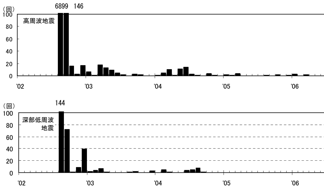
図 1※ 八丈島 月別地震回数（2002 年 8 月 13 日～2006 年 6 月 30 日）
