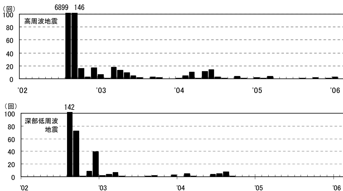
図 1※ 八丈島 月別地震回数（2002 年 8 月 13 日～2006 年 2 月 28 日）
