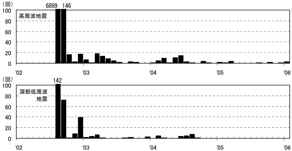
図 1 ※ 八丈島 月別地震回数（2002 年 8 月 13 日～2006 年 1 月 31 日）
