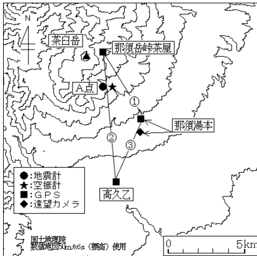
図 4 那須岳 気象庁の観測点配置図
