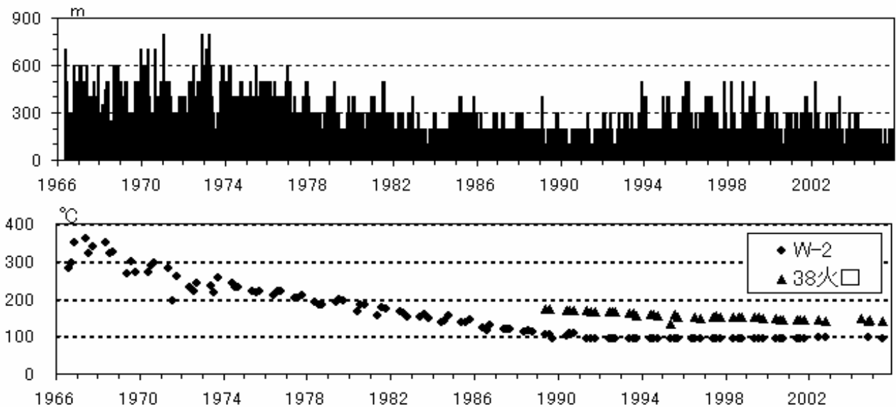
図 3 那須岳 月別最大噴煙高度 (上段) と噴気温度 (下段) (1966 年 1 月～2005 年 11 月) W-2 および 38 火口はいずれも茶臼岳西側斜面にある温度観測点
