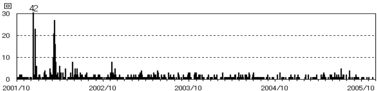
図 1 那須岳 日別地震回数 (2003 年 11 月 1 日～2005 年 11 月 30 日)
