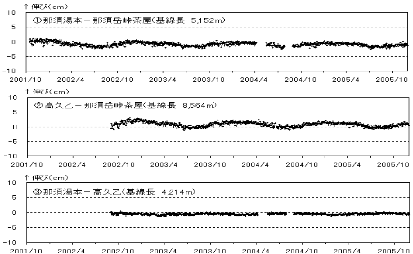
図 2 那須岳 G P S 連続観測による基線長変化 (2001 年 10 月 1 日～2005 年 11 月 30 日)
