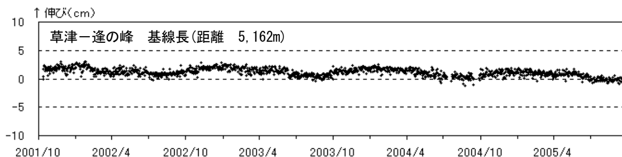
図 3 草津白根山 GPS 連続観測による基線長変化（2001 年 10 月 1 日～2005 年 9 月 30 日） その他の基線でも火山活動によるとみられる変化は観測されませんでした。
