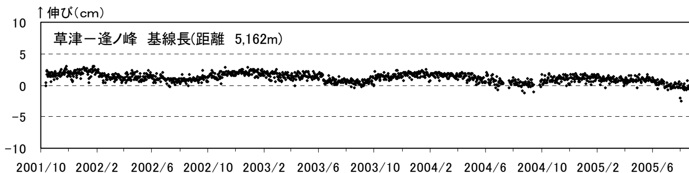
図2 草津白根山 GPS連続観測による基線長変化 (2001年10月1日～2005年8月31日) その他の基線でも火山活動によるとみられる変化は観測されませんでした。
