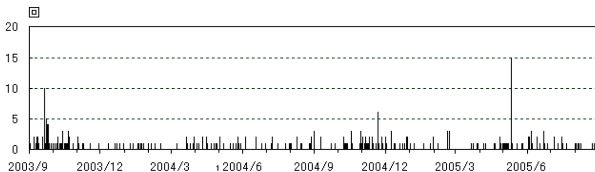
図1 草津白根山 日別地震回数 (2003年9月1日～2005年8月31日)
