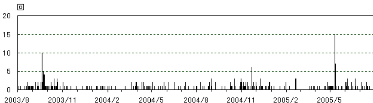
図1 草津白根山 日別地震回数（2003年8月1日～2005年7月31日） なお、今月から山体外に発生したと考えられる地震はグラフの回数から除外しています。
