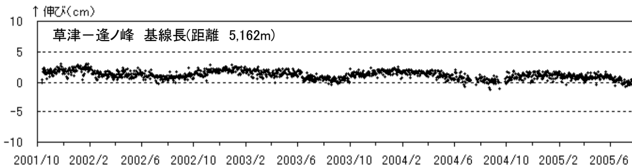
図2 草津白根山 GPS連続観測による基線長変化（2001年10月1日～2005年7月31日） その他の基線でも火山活動によるとみられる変化は観測されませんでした。
