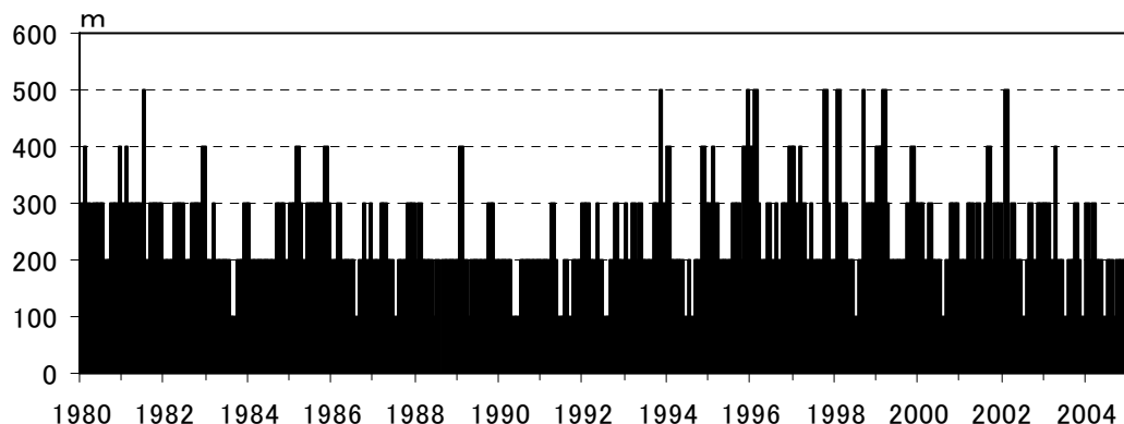
図 2 那須岳 月別最大噴煙高度（1980 年 1 月～2005 年 3 月）
