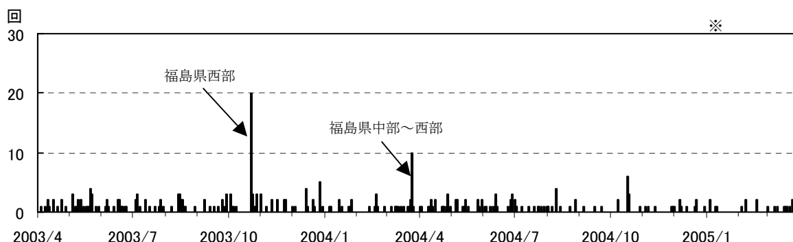
図 1 那須岳 火山性地震日別地震回数（2003 年 4 月 1 日～2005 年 3 月 31 日）
