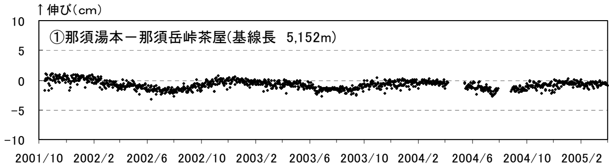
図3 那須岳 GPS観測結果(基線長変化) (2001年10月1日~2005年3月31日) その他の基線でも火山活動によるとみられる変化は観測されていない
