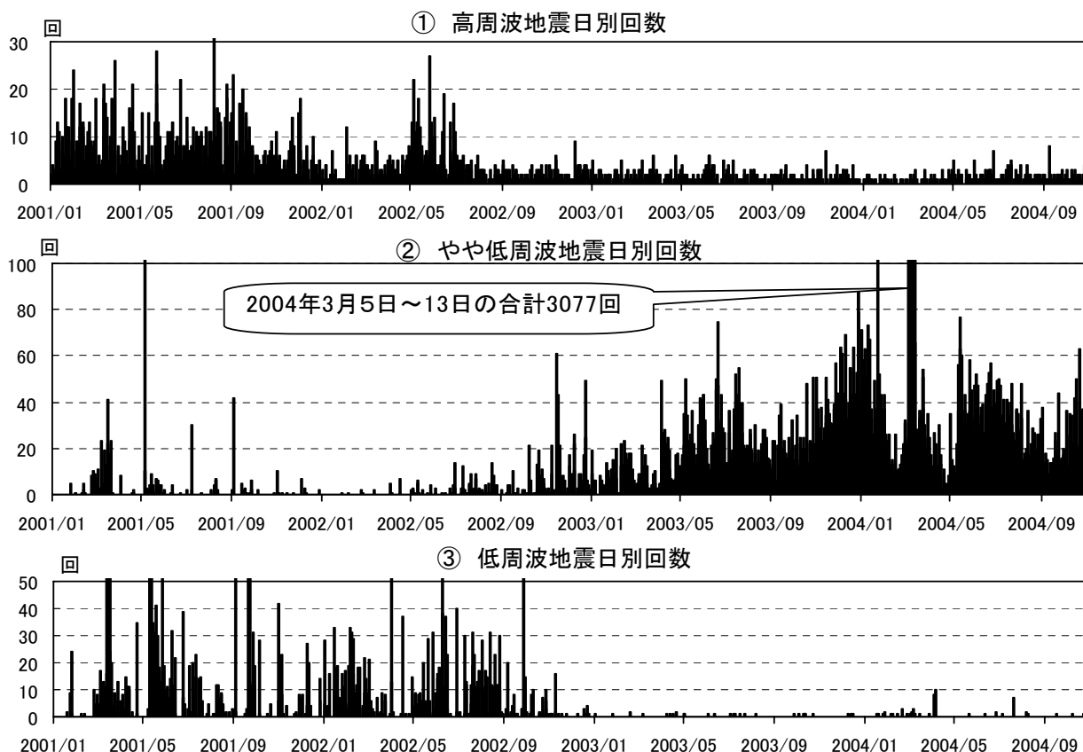
図3 三宅島 火山性地震活動経過図（2001年1月1日～2004年10月31日）
