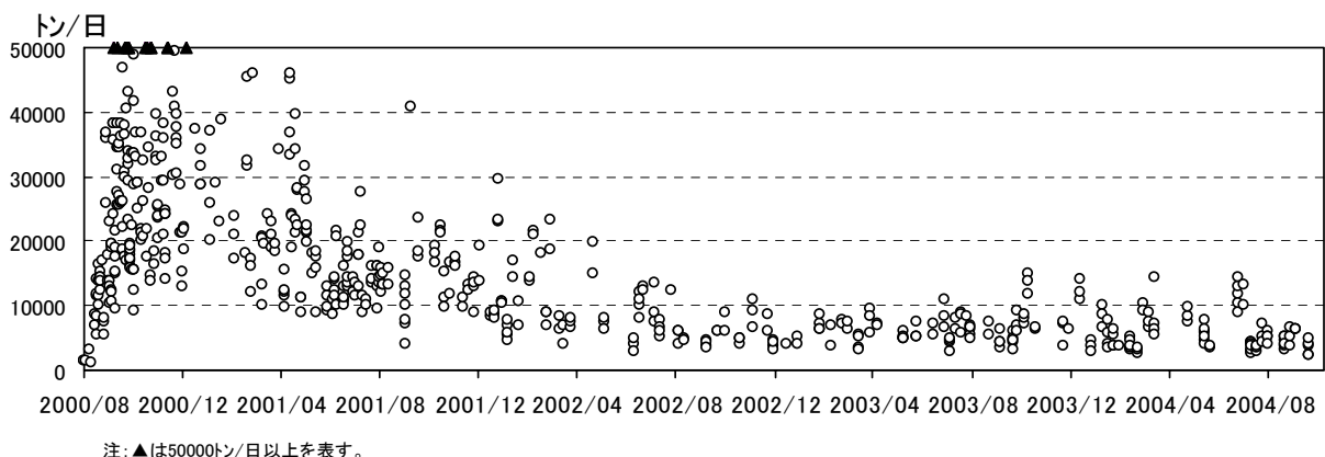
図1 三宅島 二酸化硫黄放出量(2000年8月26日～2004年10月31日)
