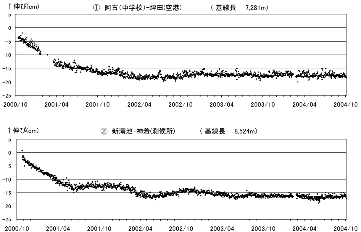
図6 三宅島 GPS観測結果(基線長変化) (2000年10月1日~2004年10月31日)
