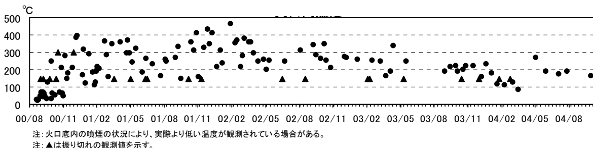
図2 三宅島 火口内温度(2000年8月26日～2004年10月31日)
