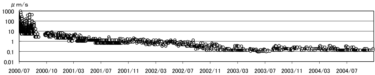
図4 三宅島 連続微動の振幅(2000年7月7日～2004年10月31日)
