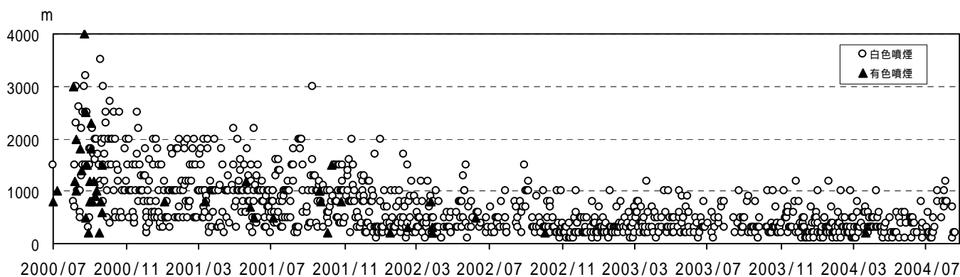
図4 三宅島 日最高噴煙高度(2000年7月8日～2004年8月31日)
