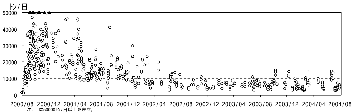
図1 三宅島 二酸化硫黄放出量(2000年8月26日~2004年8月31日)
