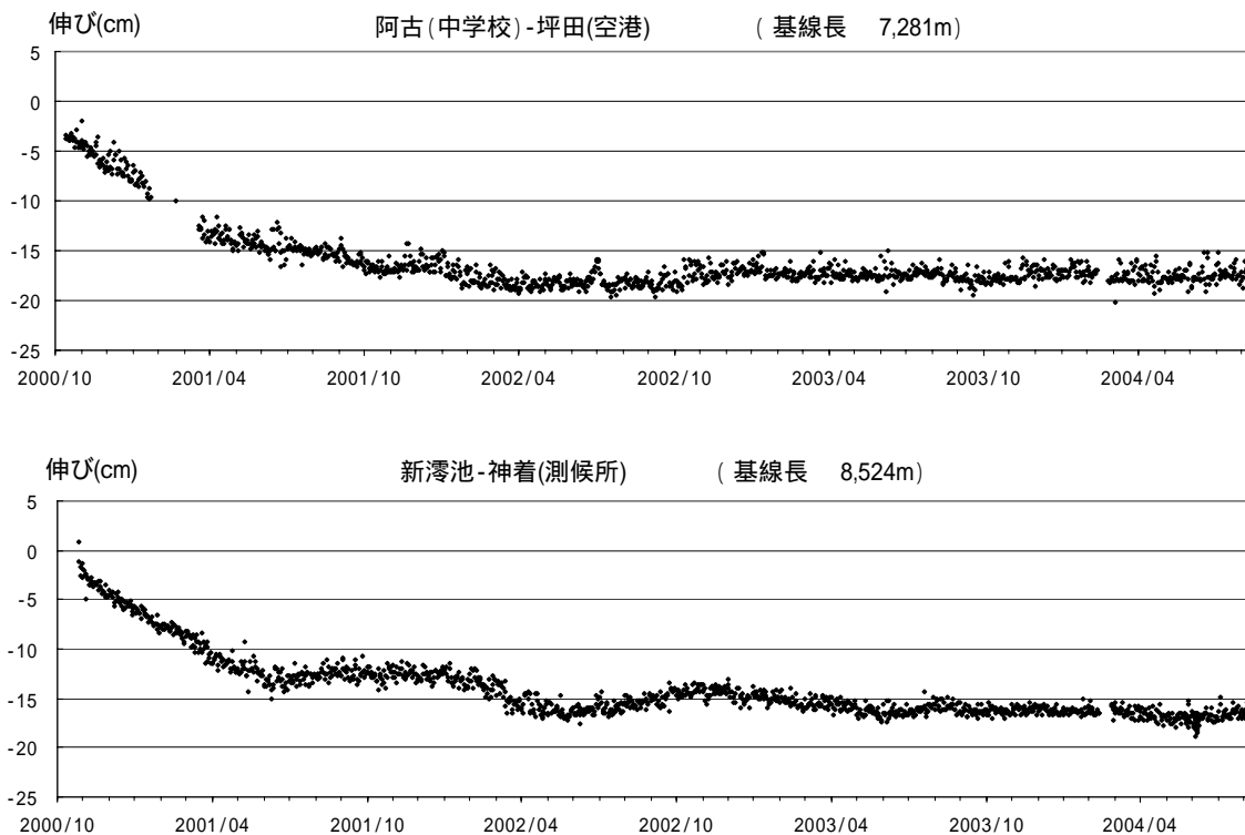
図5 三宅島 GPS観測結果(基線長変化) (2000年10月1日~2004年8月31日)
