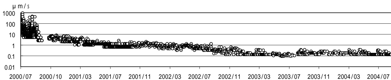
図3 三宅島 連続微動の振幅(2000年7月7日～2004年8月31日)
