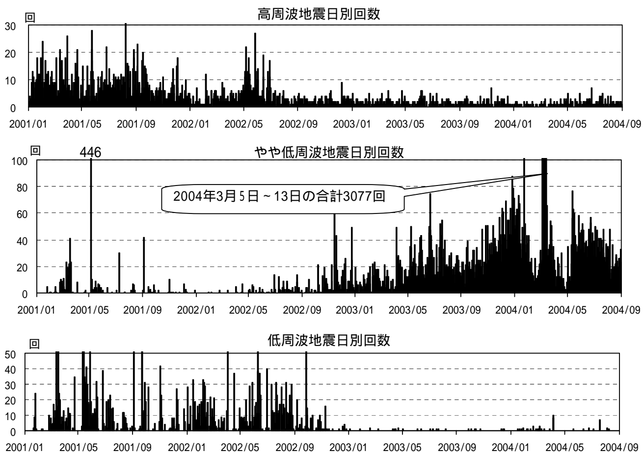
図2 三宅島 火山性地震活動経過図 (2001年1月1日～2004年8月31日)
