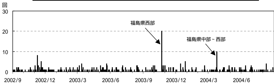
図 1 那須岳 火山性地震日別地震回数（2002 年 9 月 1 日～2004 年 8 月 31 日）
