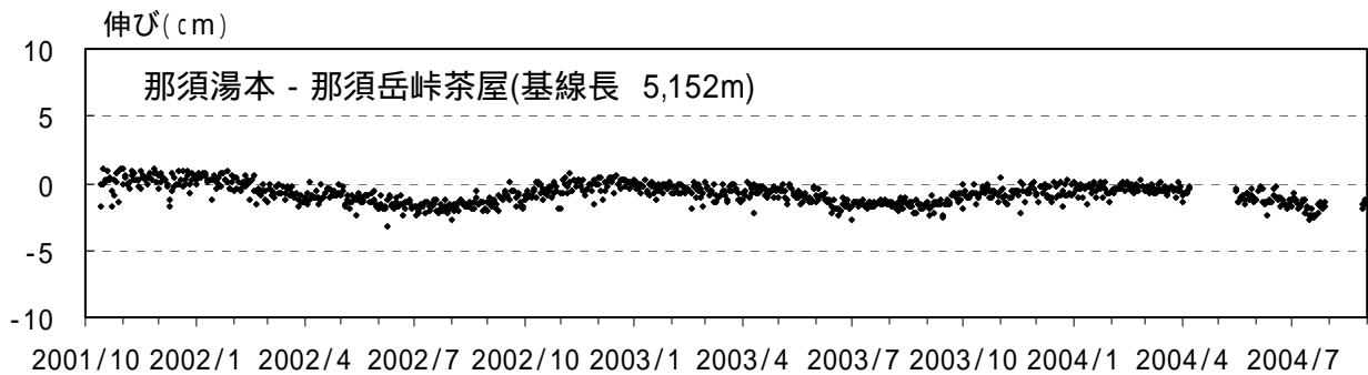
図3 那須岳 GPS観測結果(基線長変化) (2001年10月1日~2004年8月31日) その他の基線でも火山活動によると見られる変化は観測されていない
