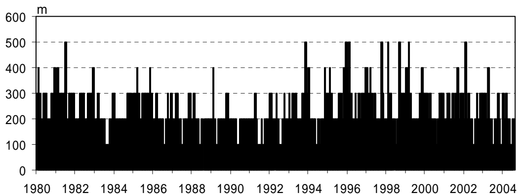
図 2 那須岳 月別最大噴煙高度（1980 年 1 月～2004 年 8 月）
