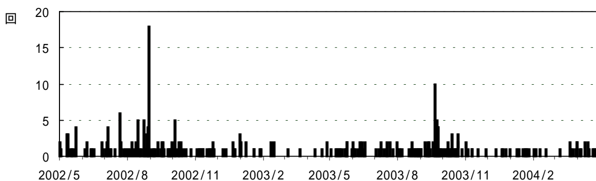
図1 草津白根山 火山性地震日別回数(2002年5月1日~2004年4月30日)
