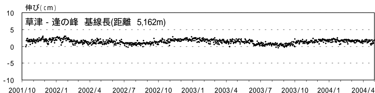
図2 草津白根山 GPS観測結果(基線長変化)(2001年10月1日~2004年4月30日)
