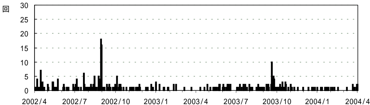
図1 草津白根山 火山性地震日別回数(2002年4月1日~2004年3月31日)
