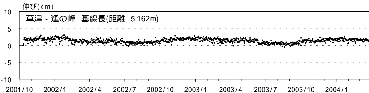
図2 草津白根山 GPS観測結果(2001年10月1日~2004年3月31日)
