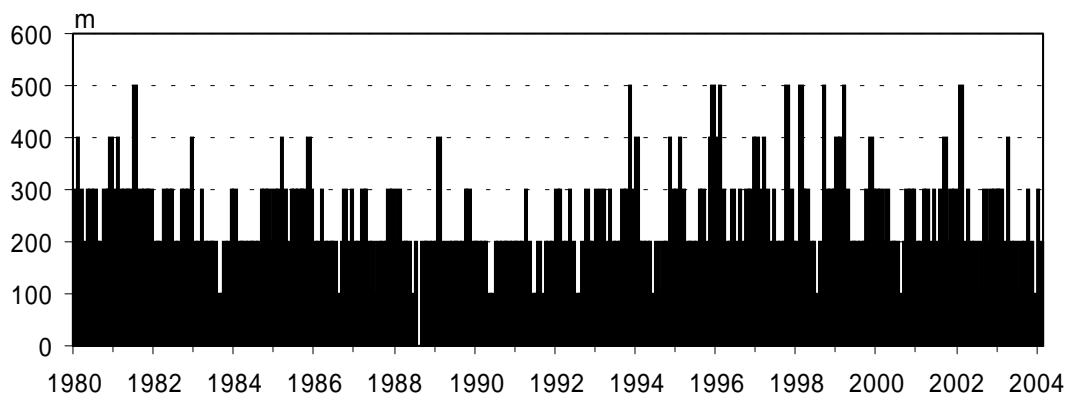
図2 那須岳 月別最高噴煙高度(1980年1月~2004年2月)
