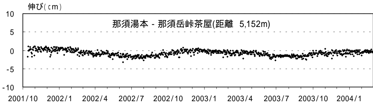
図3 那須岳 GPS観測結果(基線長変化) (2001年10月1日~2004年2月29日)
