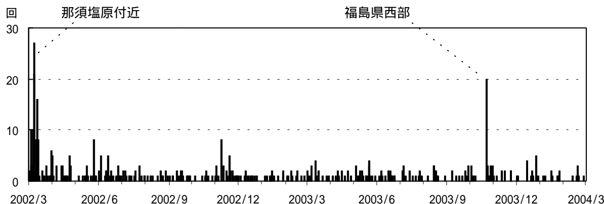
図1 那須岳 火山性地震日別回数(2002年3月1日~2004年2月29日)
