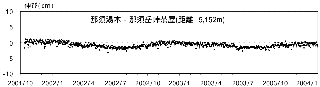
図3 那須岳 GPS 観測結果(基線長変化) (2001年10月1日~2004年1月31日)
