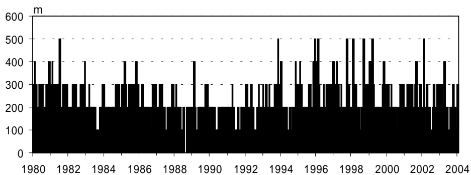
図2 那須岳 月別最高噴煙高度(1980年1月~2004年1月)
