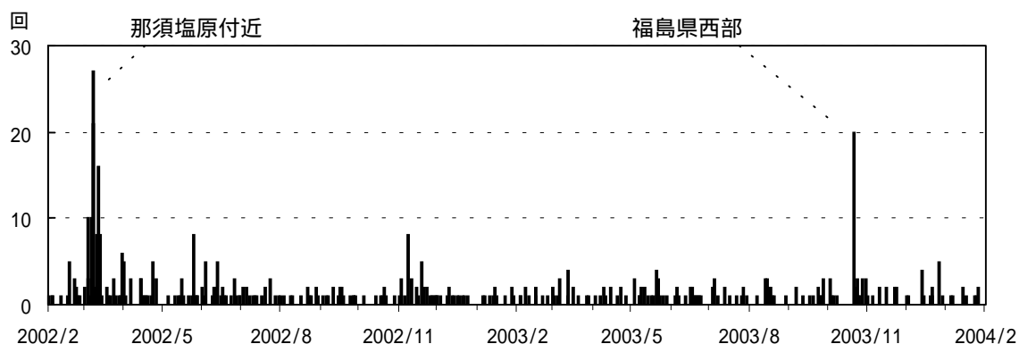
図1 那須岳 火山性地震日別回数(2002年2月1日~2004年1月31日)
