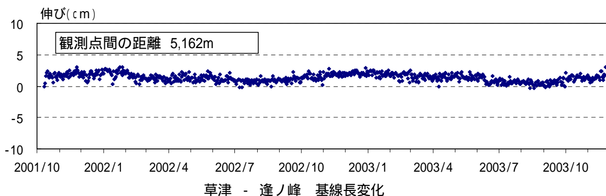
図2 草津白根山 GPS観測結果(2001年10月1日~2003年11月30日)
