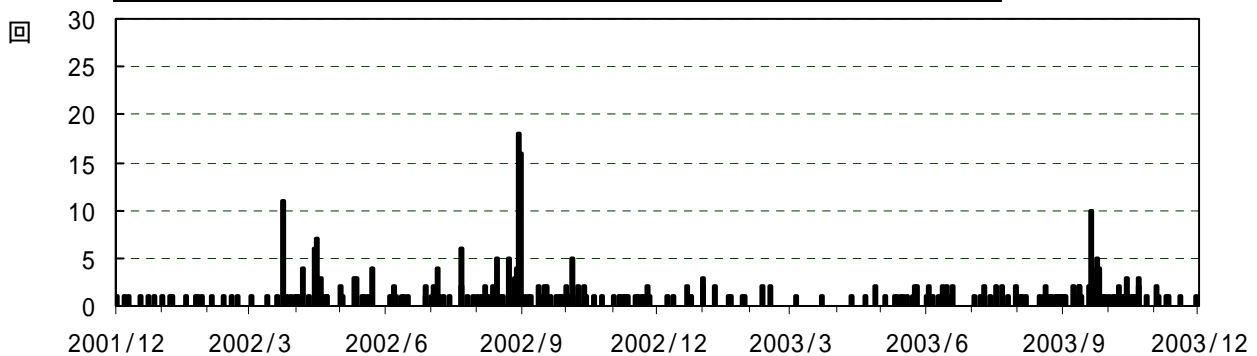
図1 草津白根山 火山性地震日別回数(2001年12月1日~2003年11月30日)
