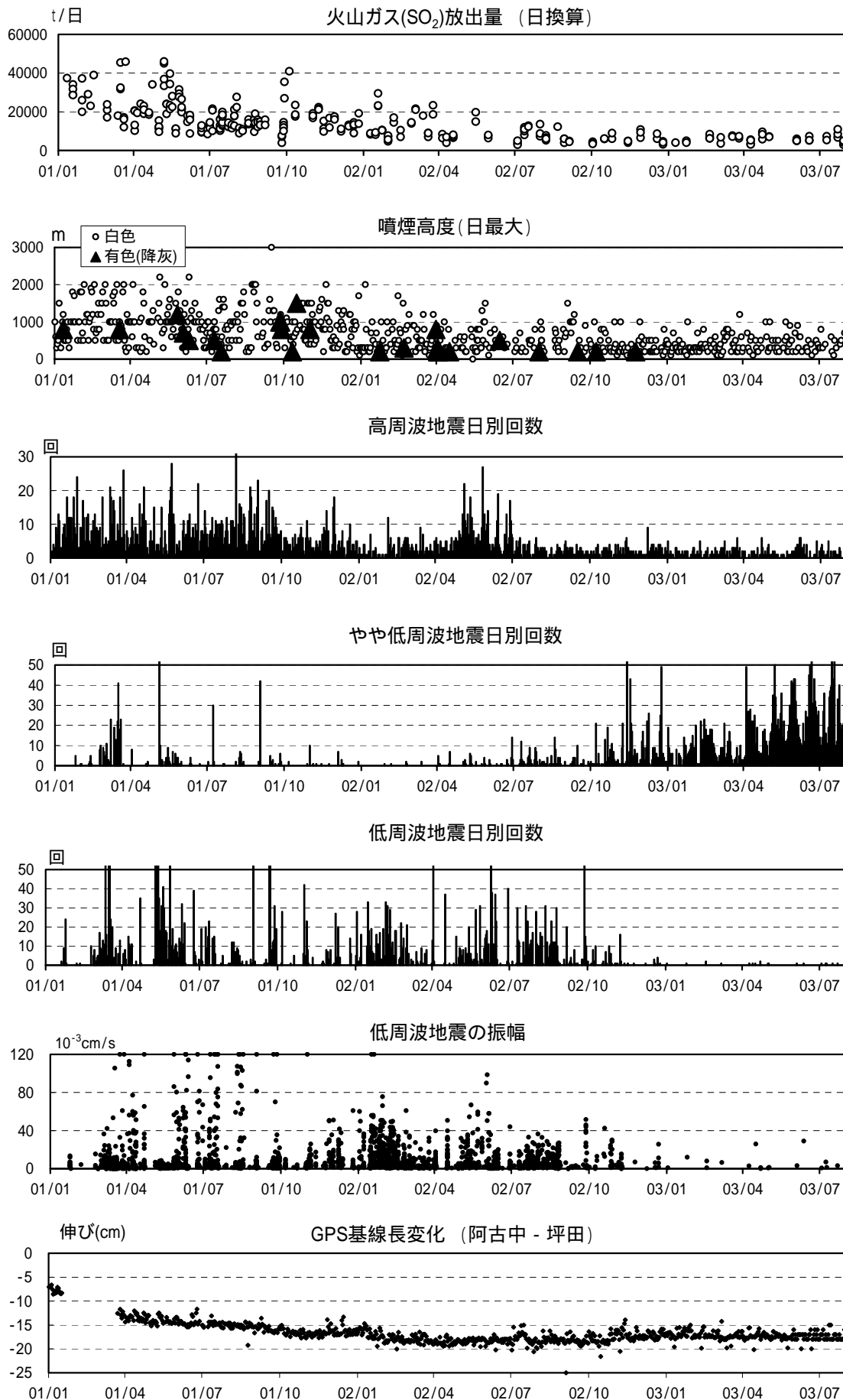
図2 三宅島火山活動経過図 (2001年1月1日~2003年7月31日)
