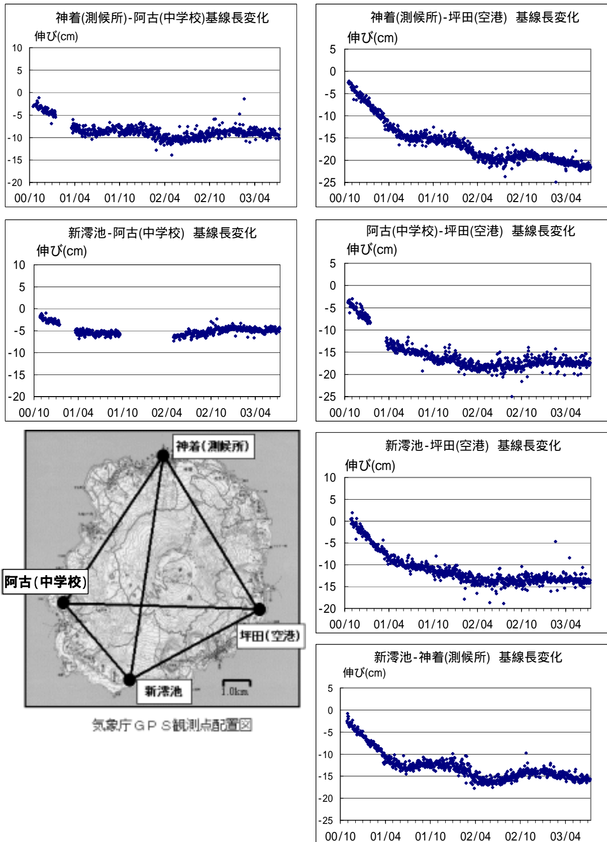
図1 三宅島GPS観測結果 (2000年10月1日~2003年7月31日)
