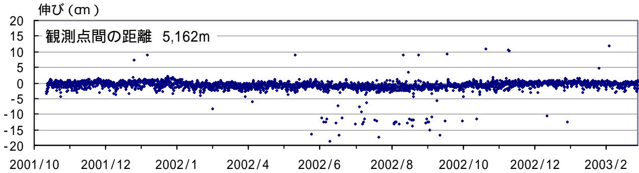
図3 草津白根山 GPS観測結果(2001年10月1日～2003年2月28日) 草津 - 逢ノ峰 基線長
