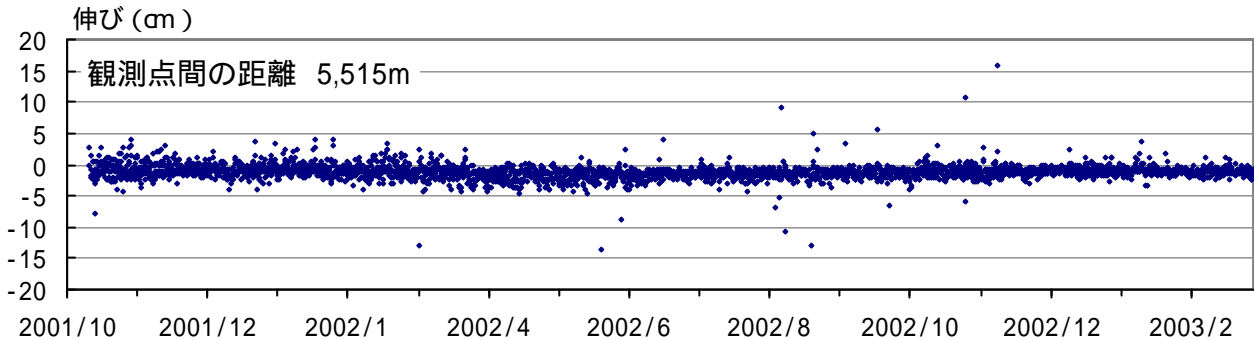
図4 草津白根山 GPS観測結果(2001年10月1日～2003年2月28日) 草津 - 仙乃入 基線長
