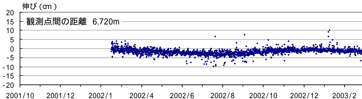
図5 草津白根山 GPS観測結果(2001年10月1日～2003年2月28日) 逢ノ峰 - 仙乃入 基線長
