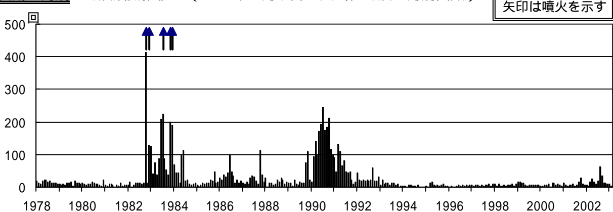
図 2 草津白根山 火山性地震月別回数及び噴火状況 (1978 年 1 月 ~ 2003 年 2 月)
