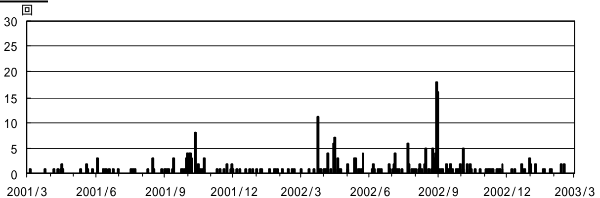
図 1 草津白根山 火山性地震日別回数 (2001 年 3 月 1 日 ~ 2003 年 2 月 28 日)
