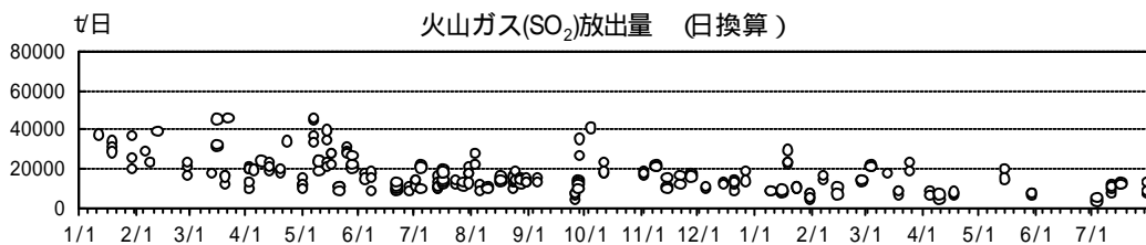
三宅島火山活動経過図 (2001年1月1日~2002年7月31日)
