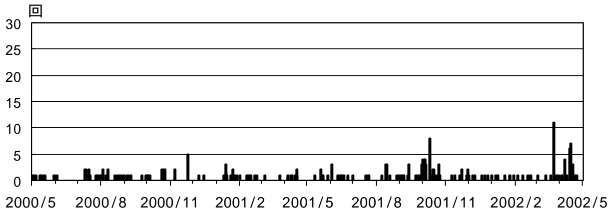
草津白根山 火山性地震日別回数表(2000年5月1日～2002年4月30日)
