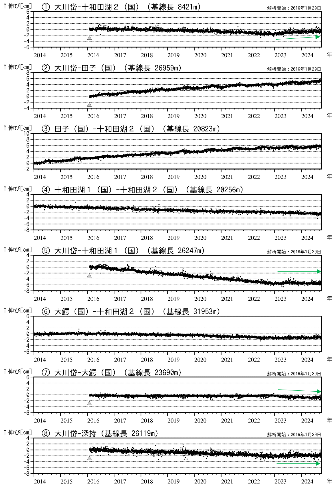
図3 十和田 GNSS 基線長変化図（2014 年 1 月～2024 年 9 月）
