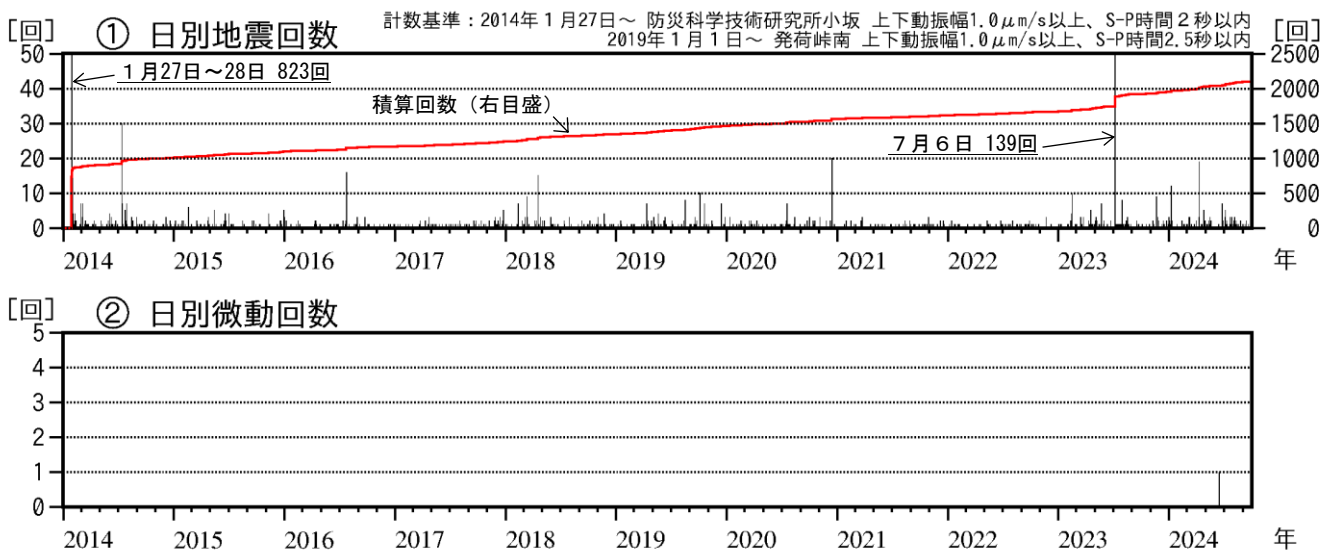
図2 十和田 活動経過図（2014年1月～2024年9月）
