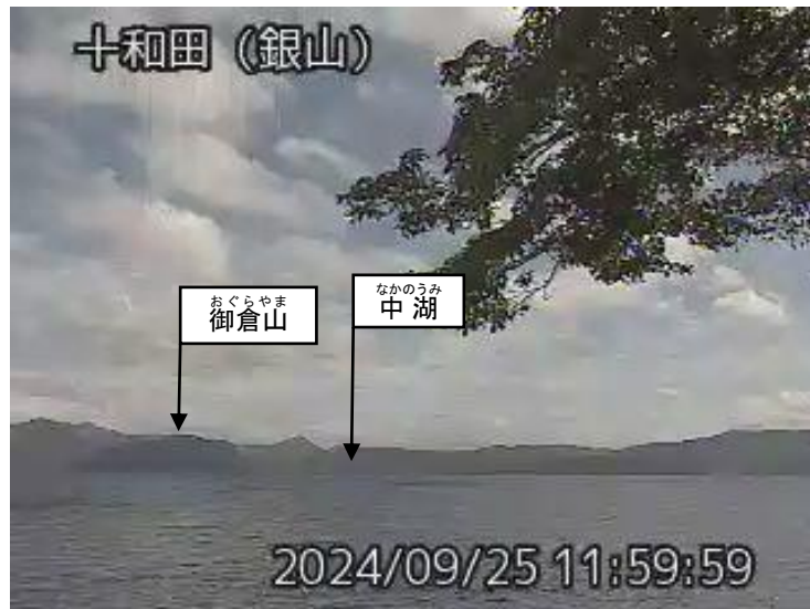
図1 十和田 中湖周辺の状況（9月25日） ・ 銀山監視カメラ（中湖の北西約6km）の映像です。
