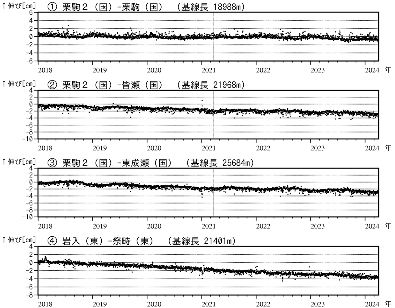
図6 栗駒山 GNSS 基線長変化図（2018年1月～2024年3月）
