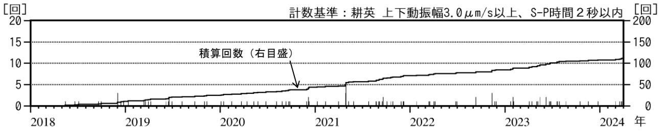
図5 栗駒山 日別地震回数（2018年1月～2024年3月）
