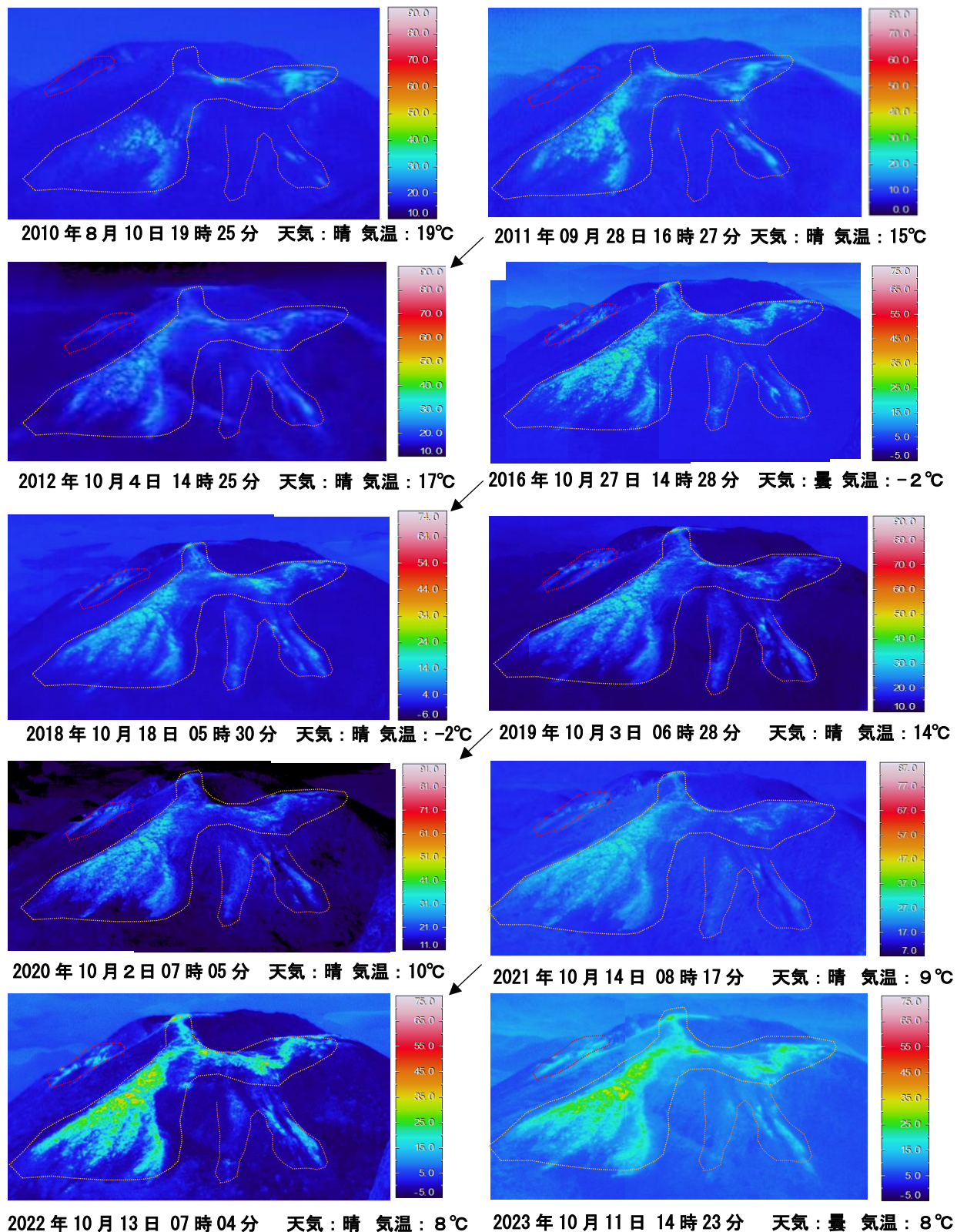
図5 秋田駒ヶ岳 北東方向から撮影した女岳の地表面温度分布の時系列変化 (2010年8月～2023年10月)
