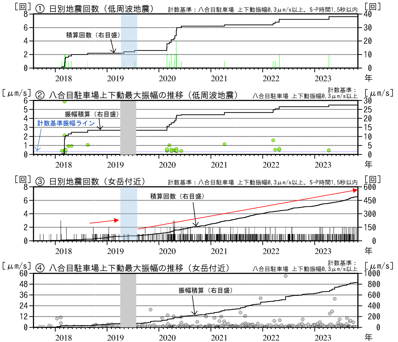
図9 秋田駒ヶ岳 低周波地震及び女岳付近の日別回数と最大振幅（2017年8月～2023年10月） ・灰色部分は八合目駐車場観測点の欠測期間を示しており、それにより地震の検知力が低下している期間を青色で示しています。
