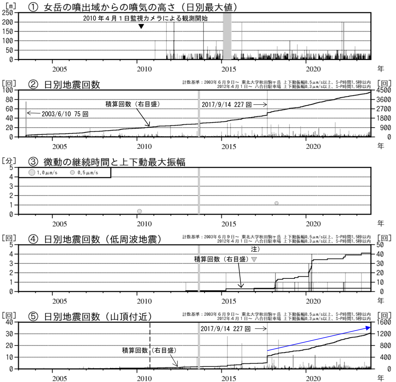
図8 秋田駒ヶ岳 火山活動経過図（2003年6月～2023年10月）
