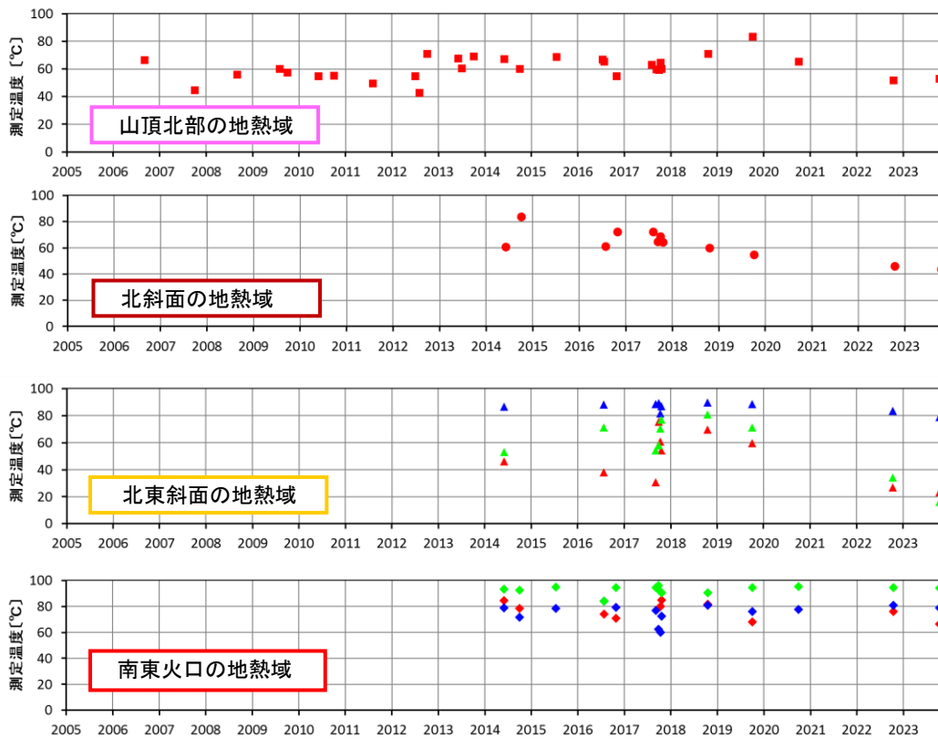
図7 女岳の地熱域における地中温度（2006年9月～2023年10月） ※測定位置は図6に対応します。
