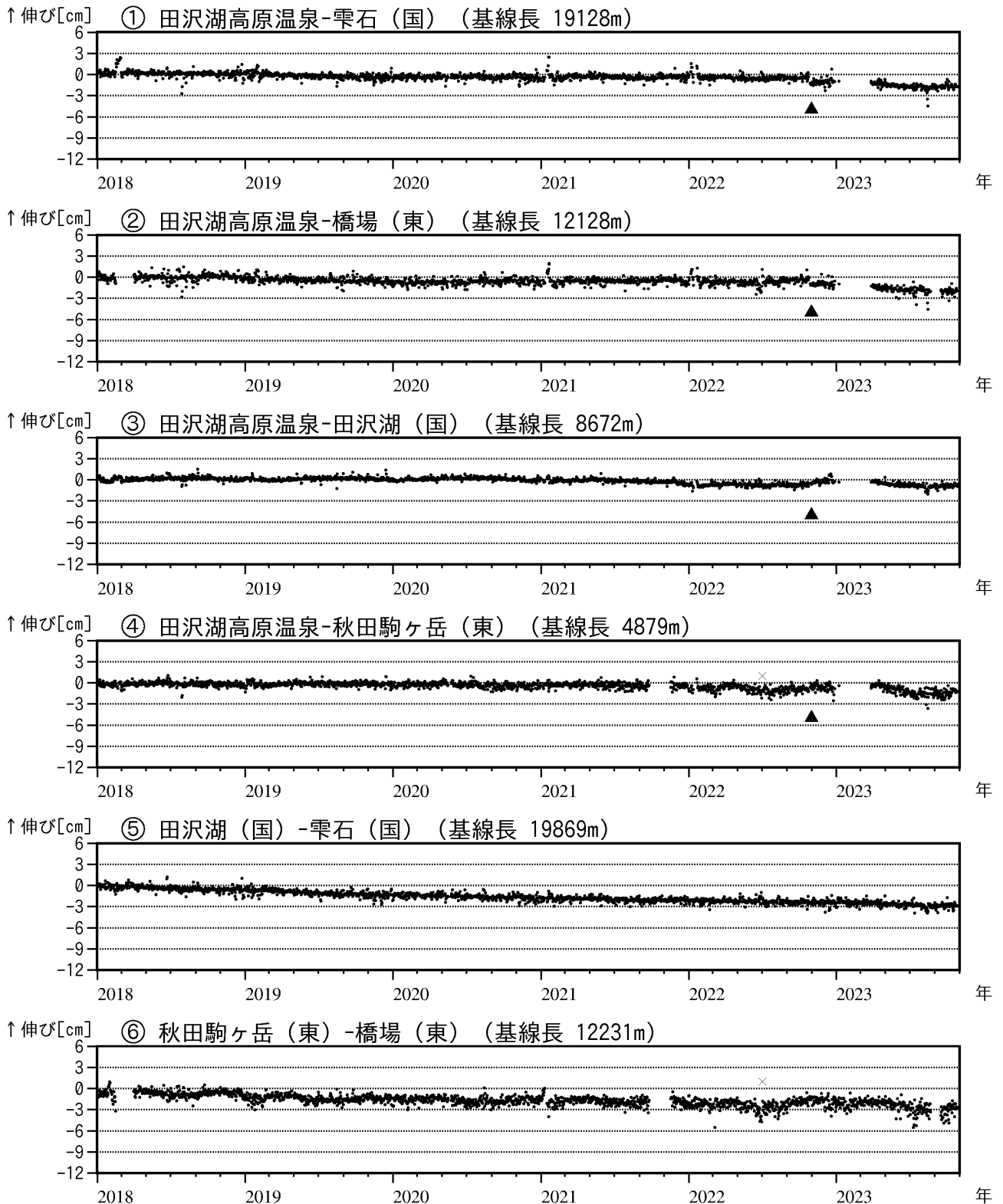
図 11 秋田駒ヶ岳 GNSS 基線長変化図 (2018 年 1 月～2023 年 10 月)
