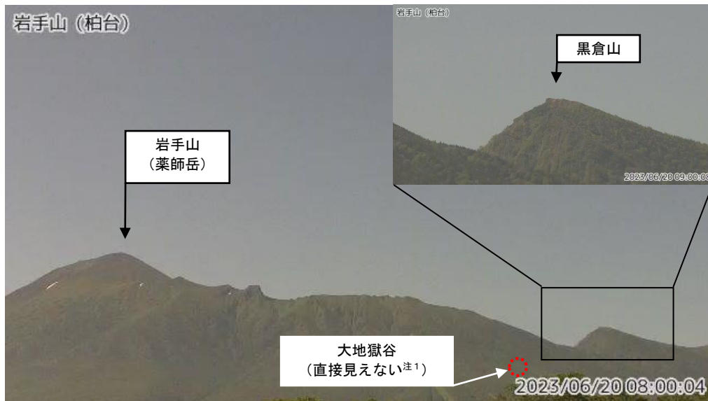
図1 岩手山 山頂部から黒倉山周辺の状況（6月20日）
