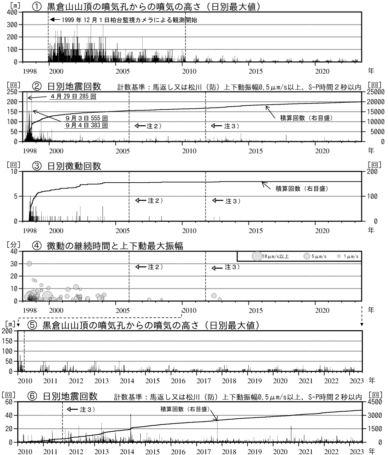
図3 岩手山 火山活動経過図（1998年1月～2023年6月）
