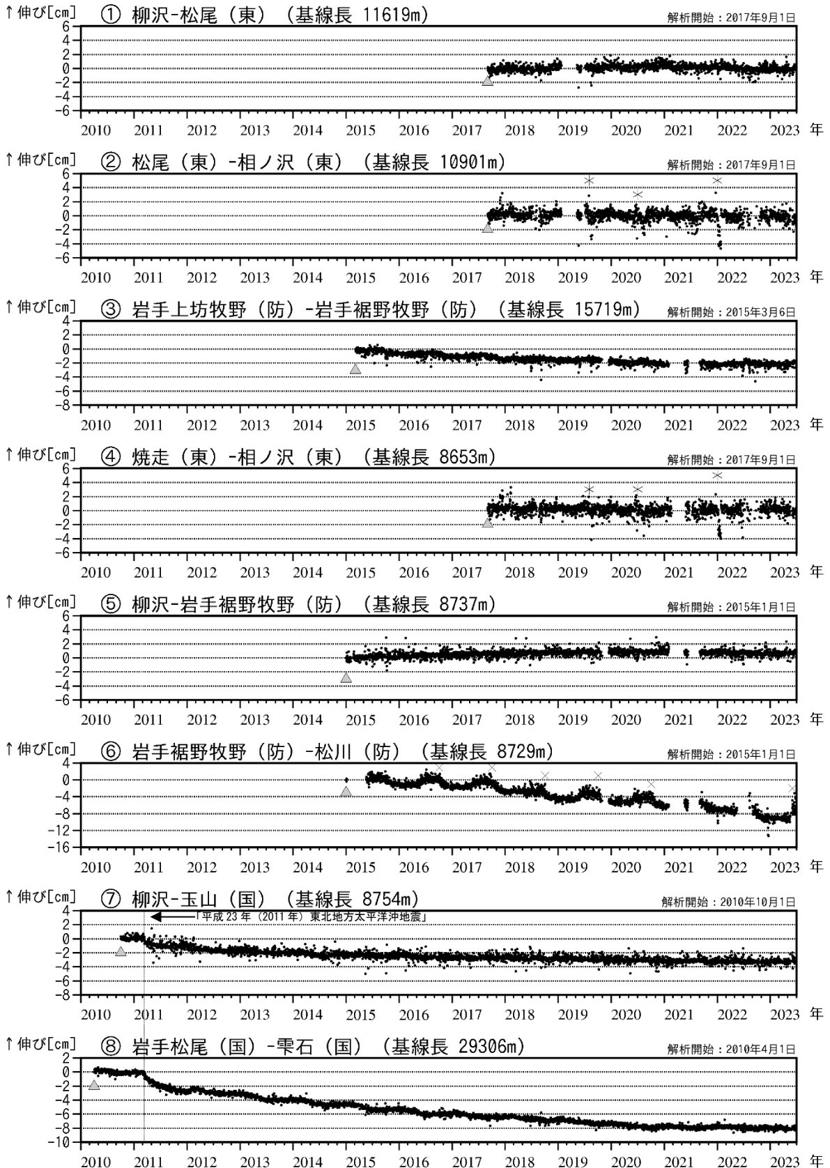
図4 岩手山 GNSS 基線長変化図（2010年4月～2023年6月）
