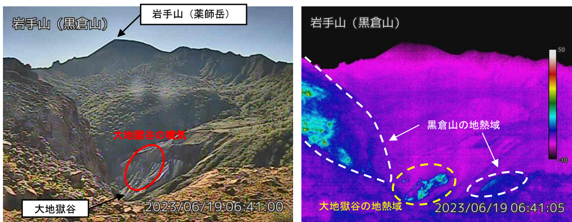
図2 岩手山 黒倉山監視カメラからの状況と地表面温度分布（6月19日）
