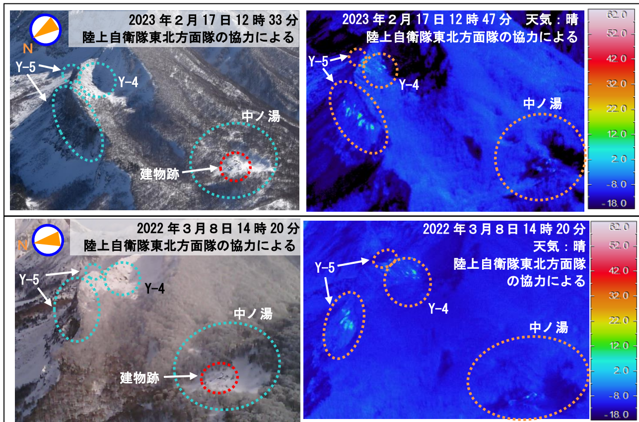
図6 磐梯山 上空から撮影した山体北側火口壁噴気地帯（Y-4、Y-5）及び中ノ湯の状況と地表面温度分布
