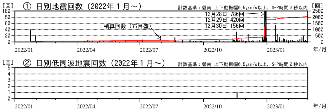
図8 磐梯山 地震回数（2022年1月～2023年2月）
