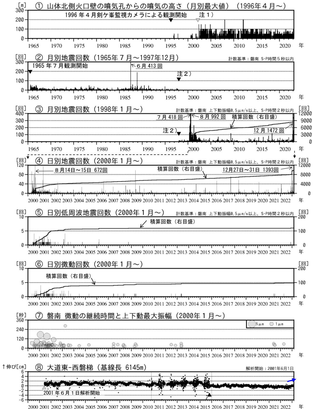
図7 磐梯山 火山活動経過図（1965年7月～2023年2月）
