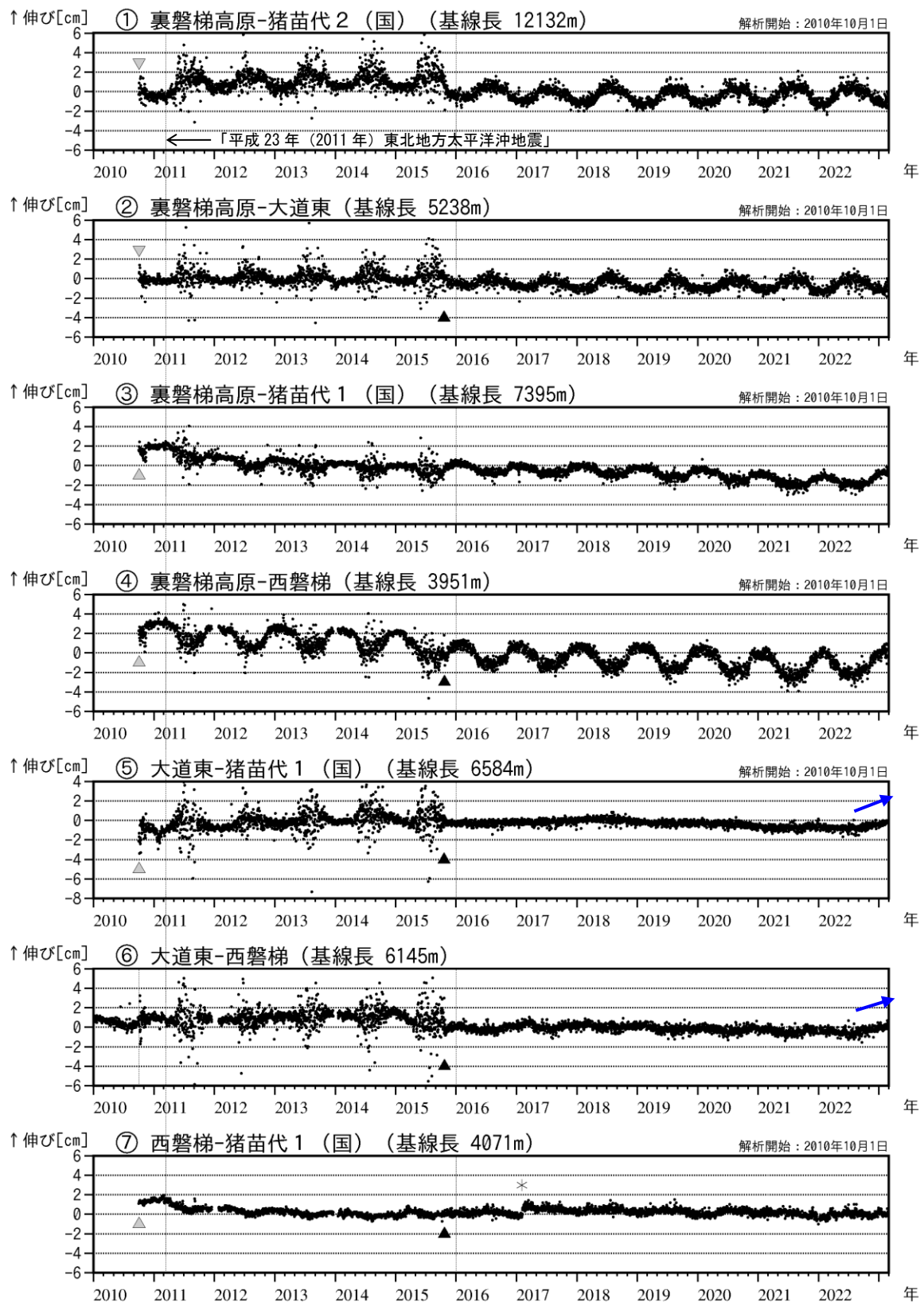
図10 磐梯山 GNSS 基線長変化図 (2010年1月～2023年2月)
