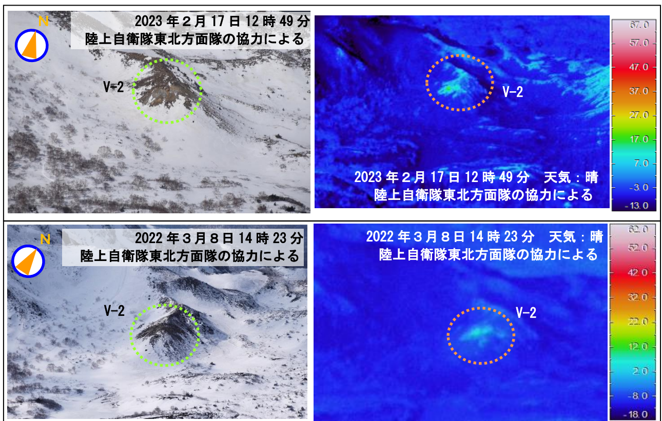
図4 磐梯山 上空から撮影した沼ノ平(V-2)の状況と地表面温度分布
