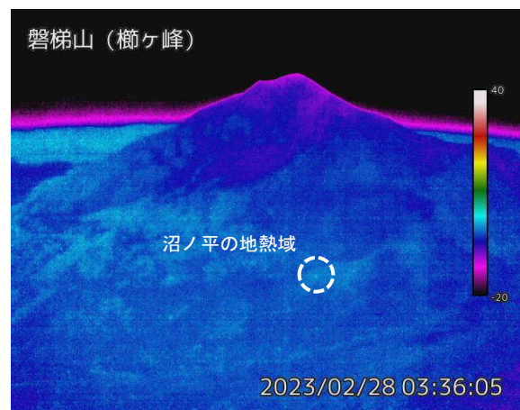
図2 磐梯山 沼ノ平周辺の状況と地表面温度分布（2月28日）
