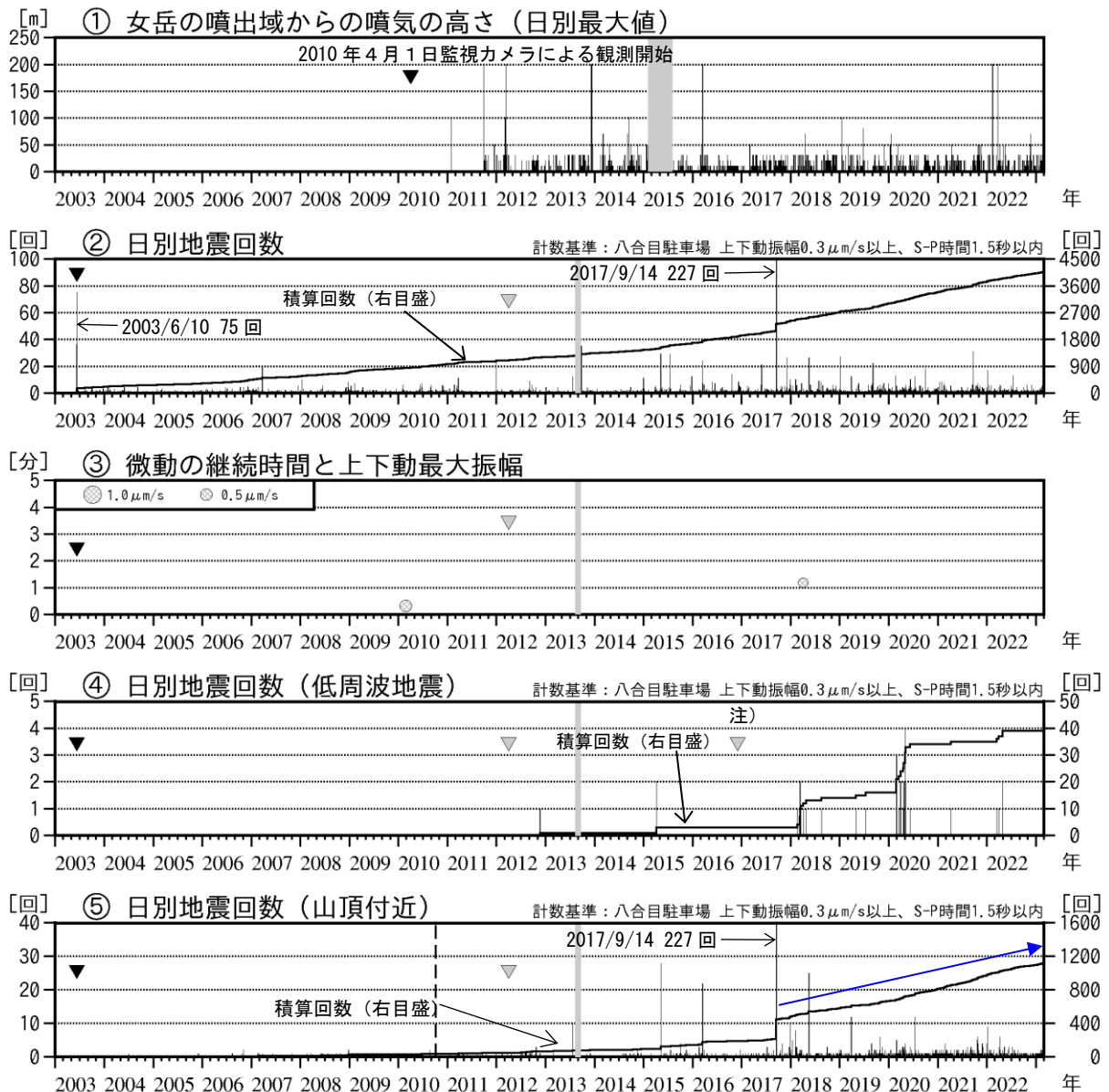
図4 秋田駒ヶ岳 火山活動経過図（2003年6月～2023年2月）
