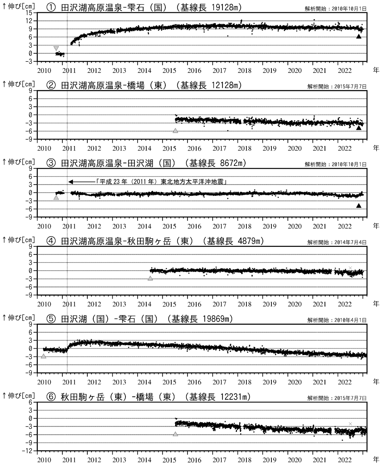
図7 秋田駒ヶ岳 GNSS 基線長変化図（2010年4月～2023年2月）
