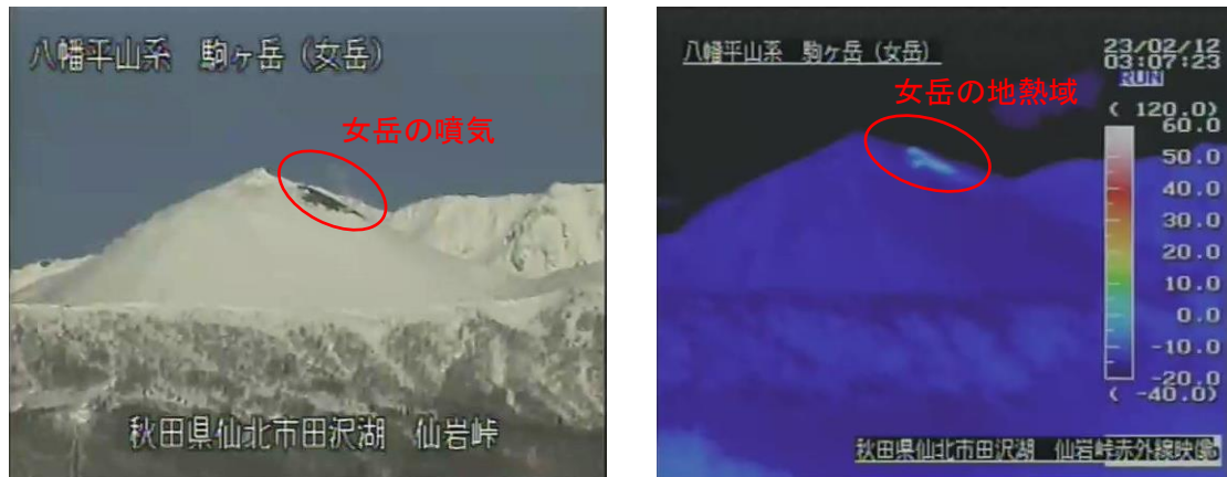
図1 秋田駒ヶ岳 女岳周辺の噴気と地表面温度分布の状況（可視：2月11日、赤外：2月12日） ・東北地方整備局が設置している仙岩峠監視カメラ（女岳山頂の南約5km）の可視及び赤外映像です。
