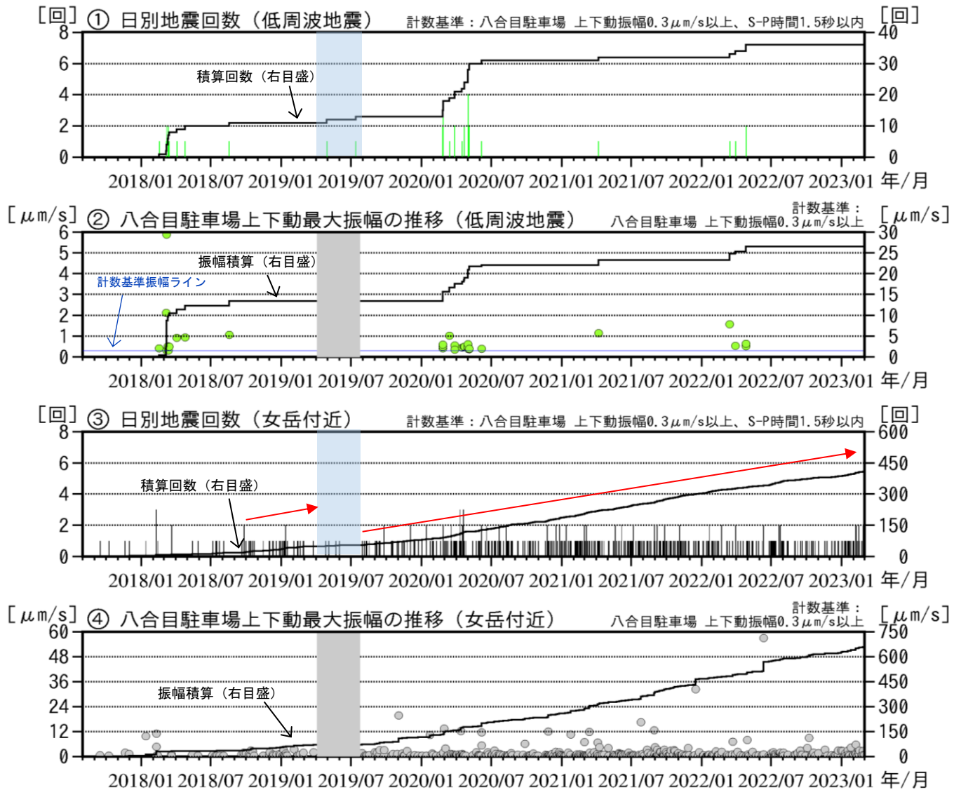
図5 秋田駒ヶ岳 低周波地震及び女岳付近の日別回数と最大振幅（2017年8月～2023年2月）
