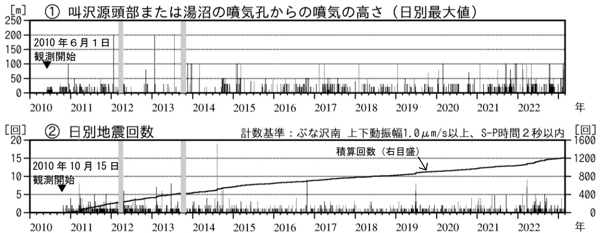
図7 秋田焼山 火山活動経過図（2010年6月～2023年2月）
