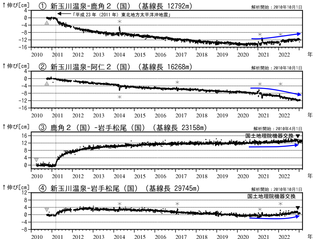
図8 秋田焼山 GNSS 基線長変化図（2010年4月～2023年2月）
