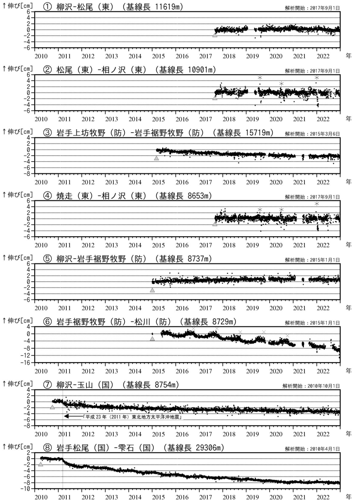
図4 岩手山 GNSS 基線長変化図 (2010年4月～2022年12月)
