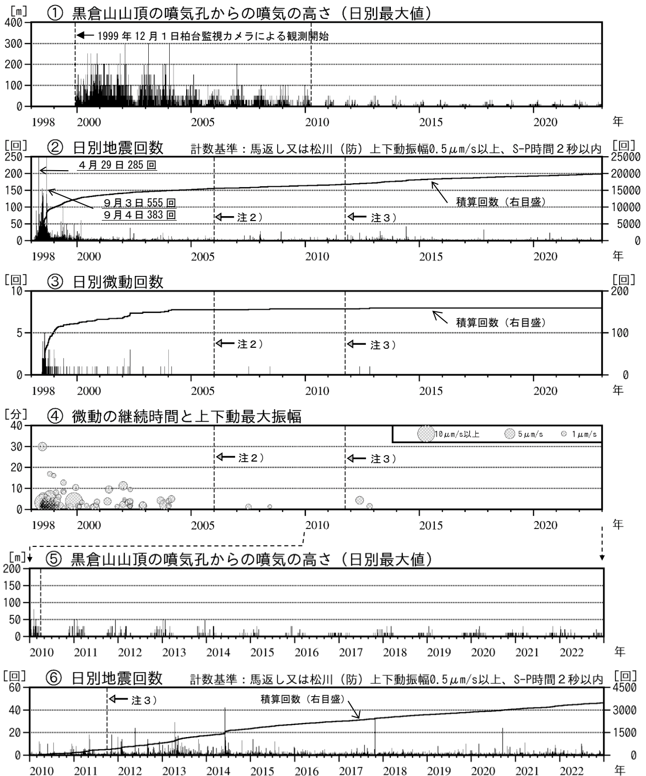
図3 岩手山 火山活動経過図（1998年1月～2022年12月）
