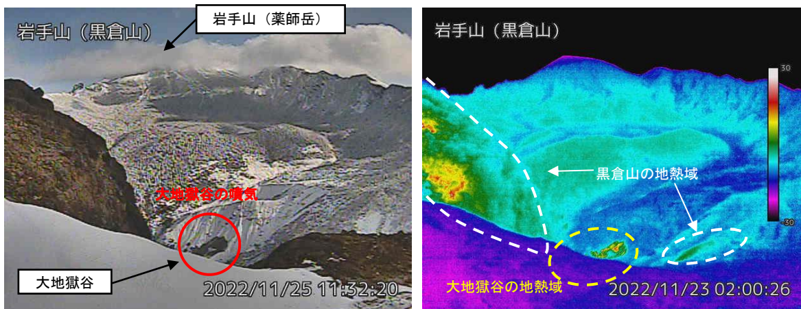
図2 岩手山 黒倉山監視カメラからの状況（11月25日）と地表面温度分布（11月23日）
