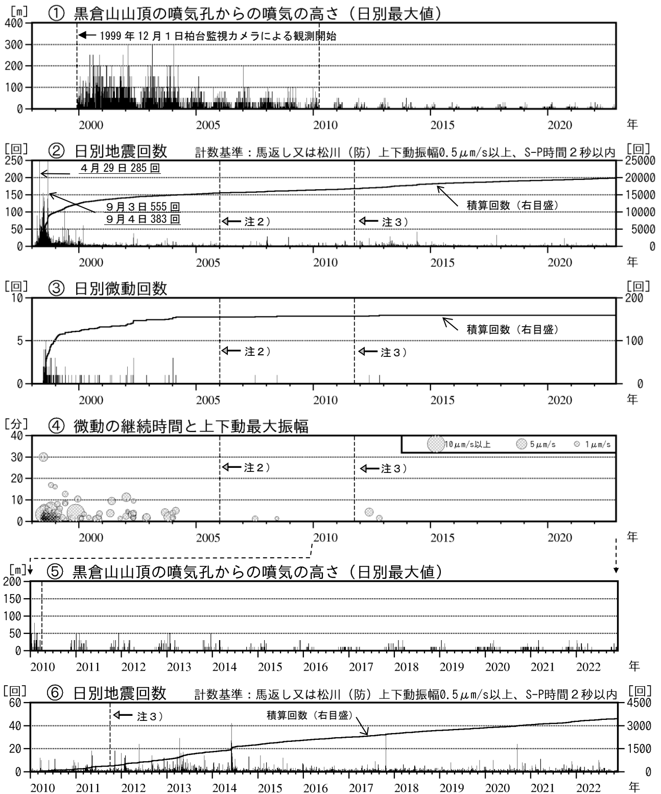
図3 岩手山 火山活動経過図（1998年1月～2022年11月）
