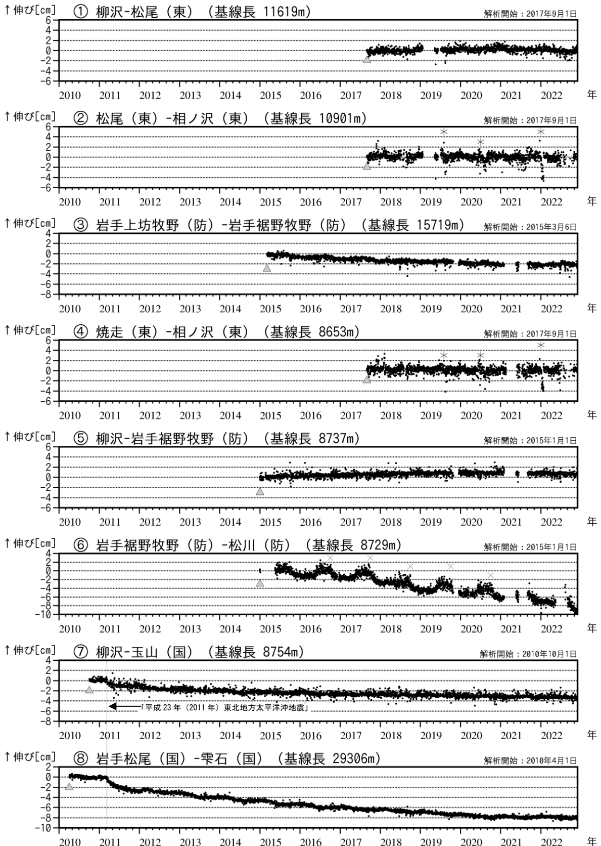
図4 岩手山 GNSS 基線長変化図 (2010年4月~2022年11月)
