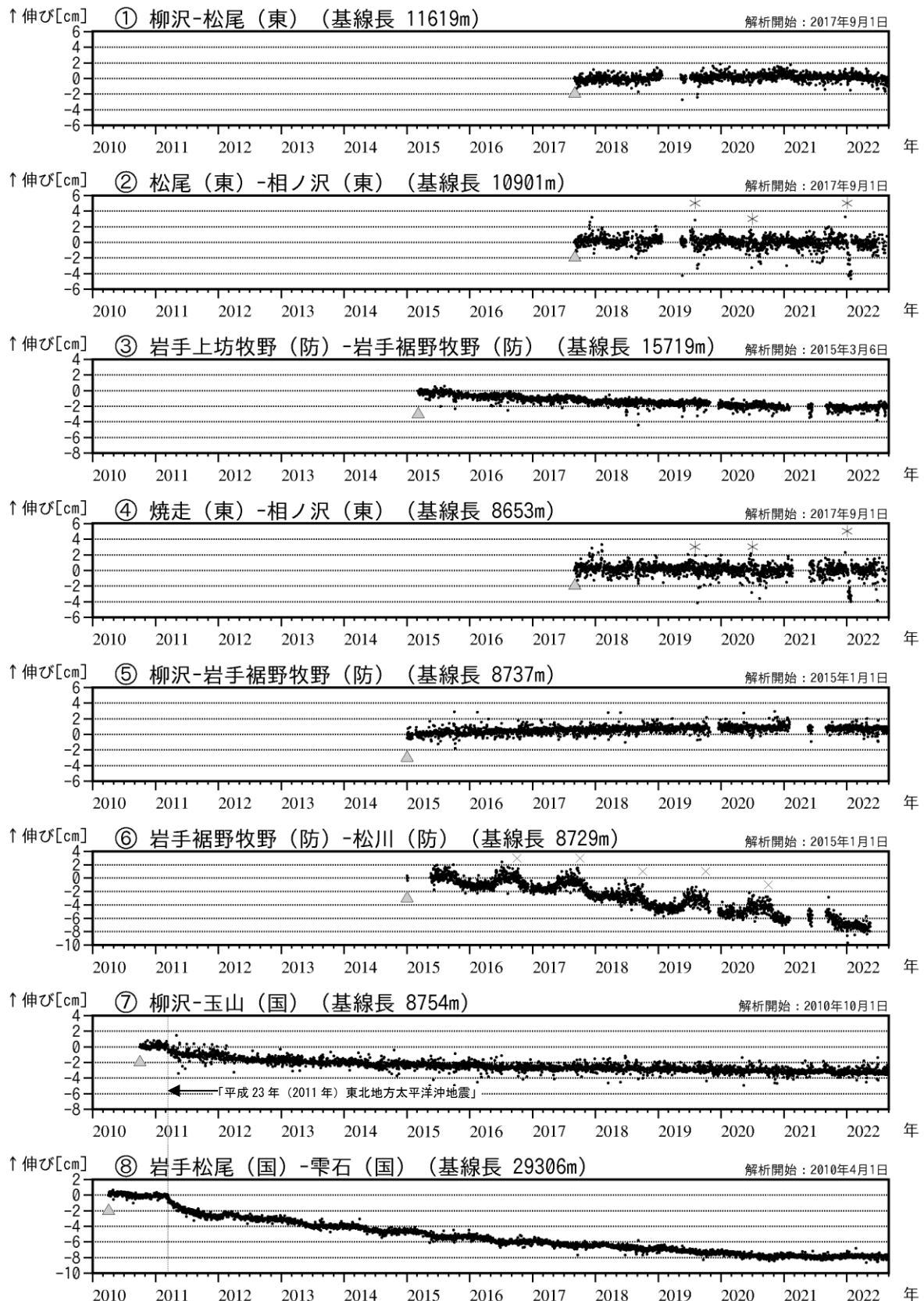
図4 岩手山 GNSS 基線長変化図 (2010年4月~2022年8月)
