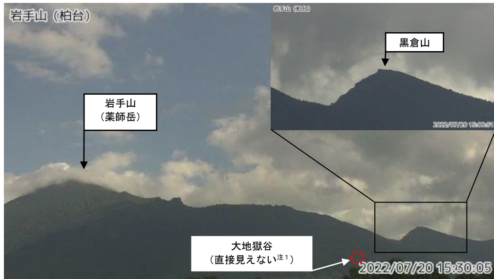
図1 岩手山 山頂部から黒倉山周辺の状況（7月20日）
