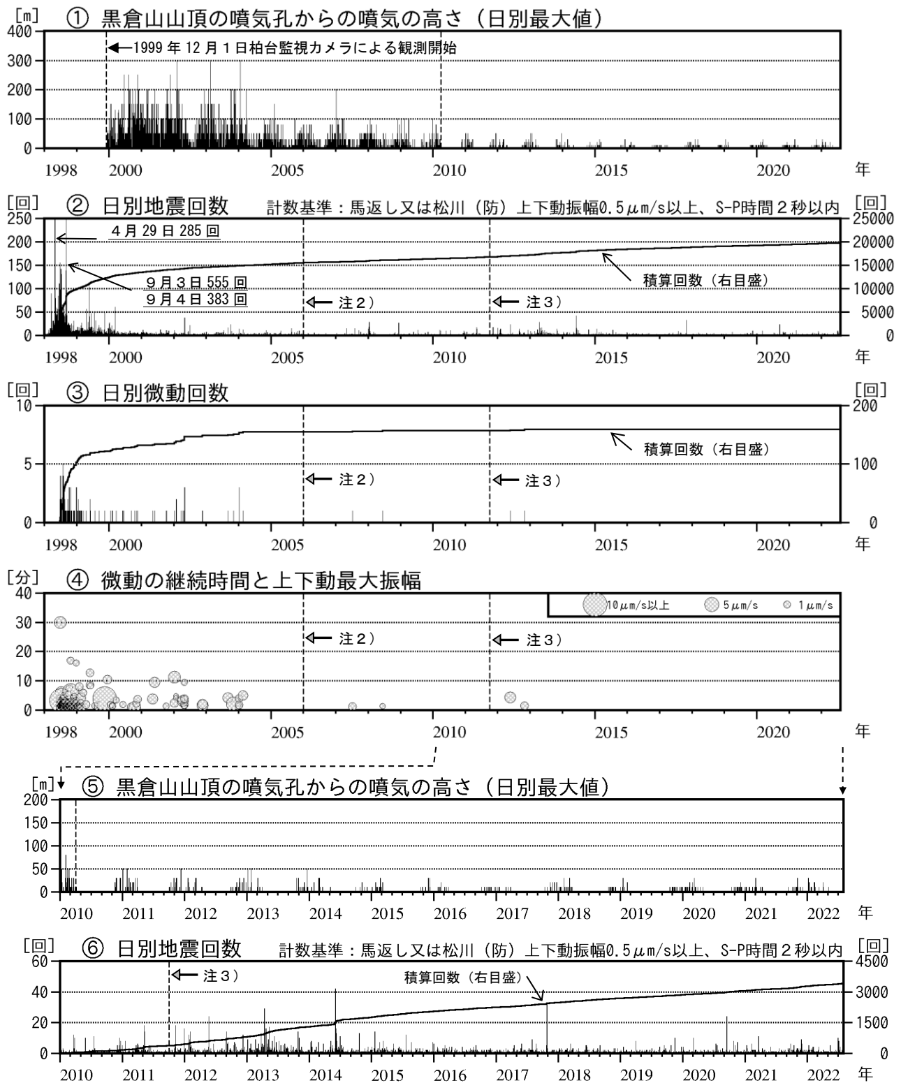
図3 岩手山 火山活動経過図（1998年1月～2022年7月）
