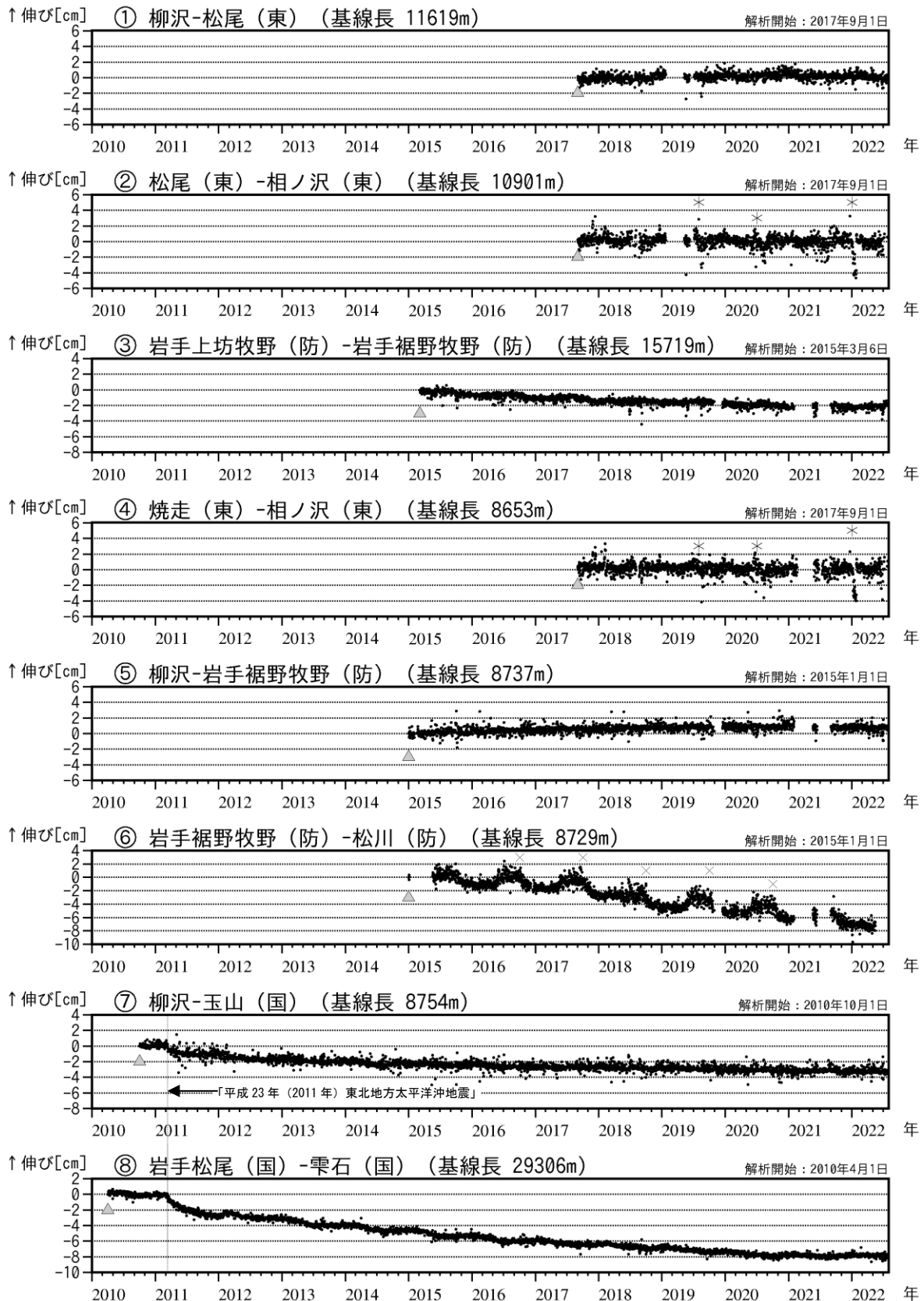
図4 岩手山 GNSS 基線長変化図 (2010年4月~2022年7月)
