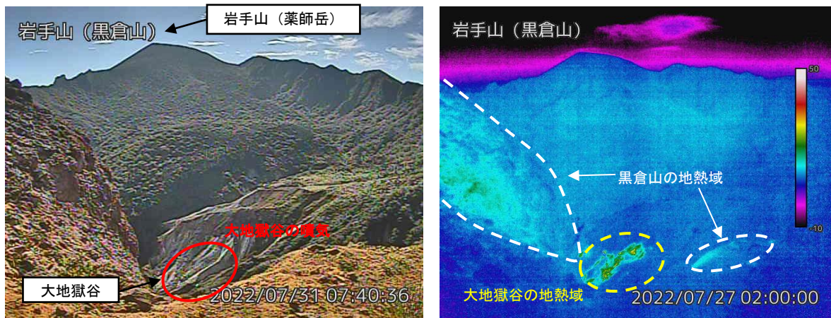
図2 岩手山 黒倉山監視カメラからの状況（7月31日）と地表面温度分布（7月27日）
