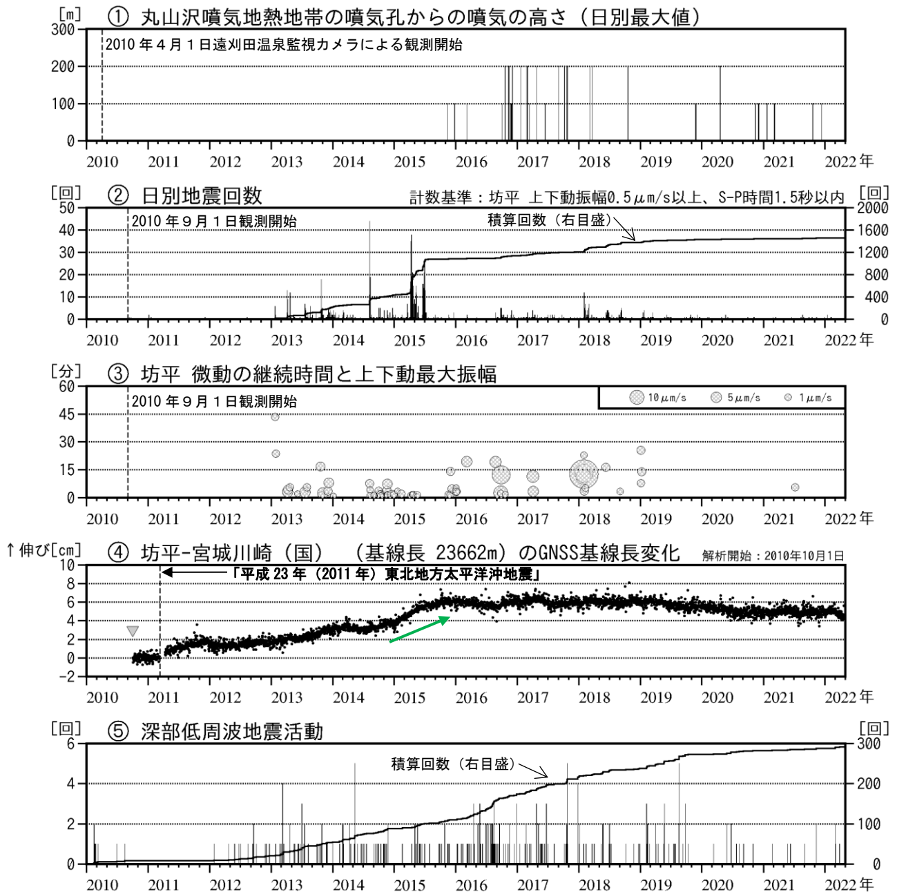
図2 蔵王山 火山活動経過図（2010年4月～2022年4月）
