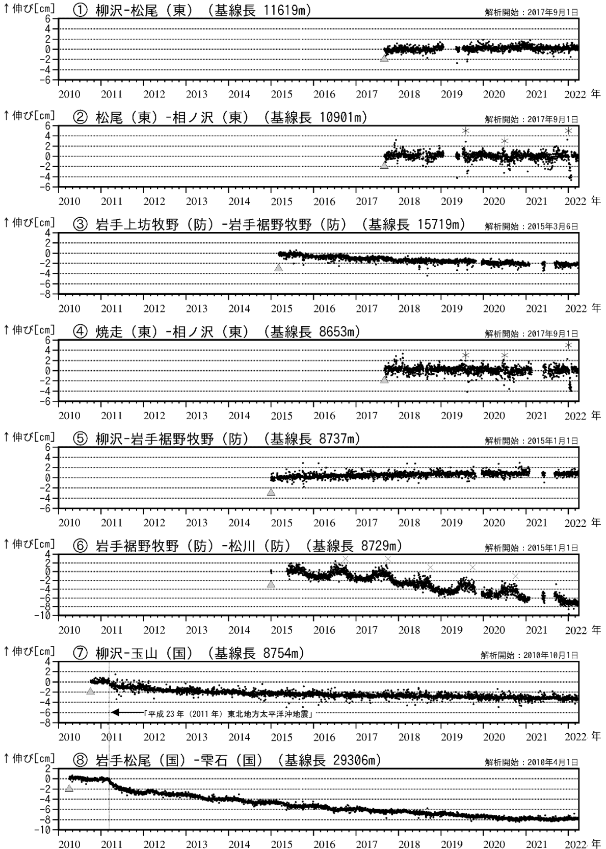
図7 岩手山 GNSS 基線長変化図（2010年4月～2022年3月）
