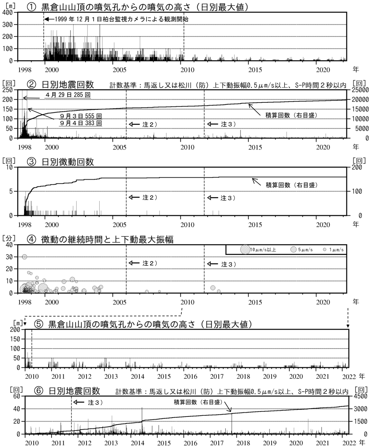
図6 岩手山 火山活動経過図（1998年1月～2022年3月）
