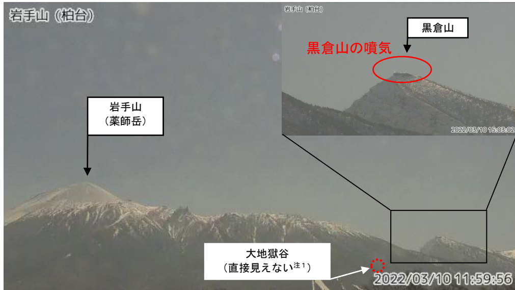
図1 岩手山 山頂部から黒倉山周辺の状況（3月10日）
