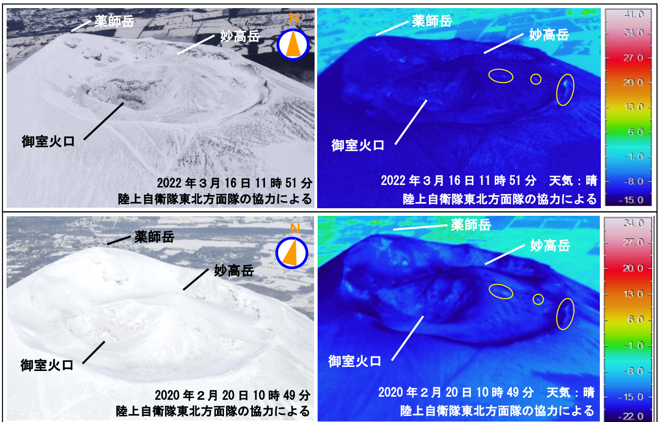
図5 岩手山 上空からの岩手山山頂の状況と地表面温度分布
