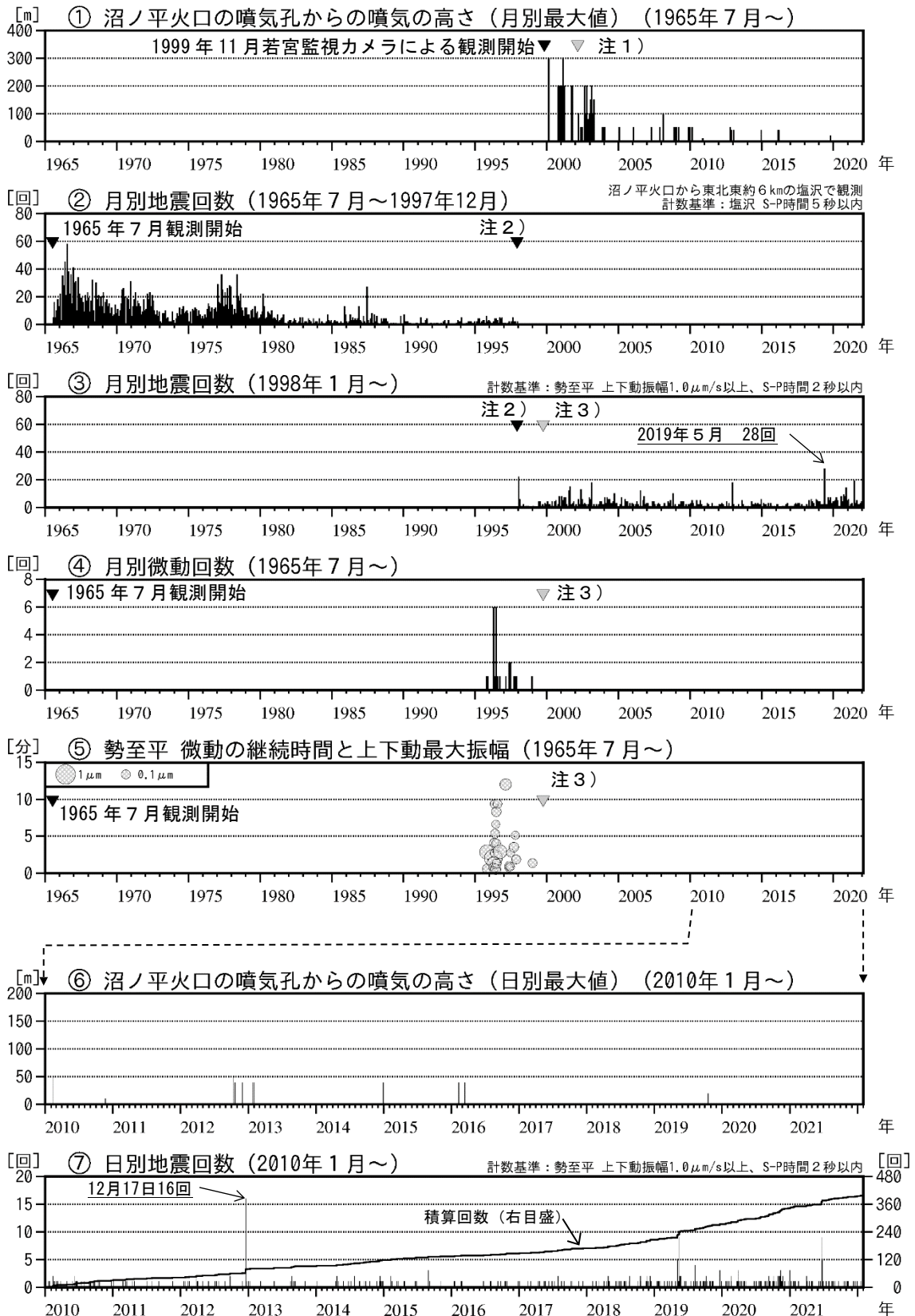
図2 安達太良山 火山活動経過図（1965年7月～2022年1月）
