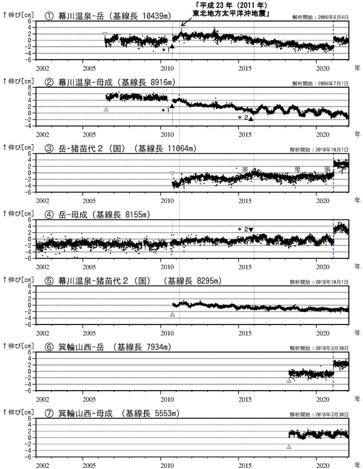
図3 安達太良山 GNSS 基線長変化図（2002年1月～2022年1月）
