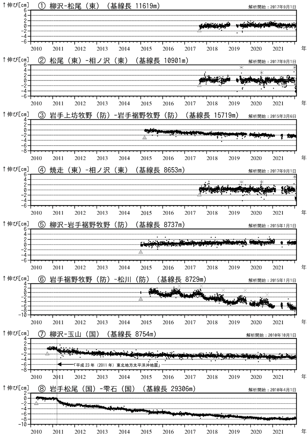
図3 岩手山 GNSS 基線長変化図 (2010年4月～2022年1月)
