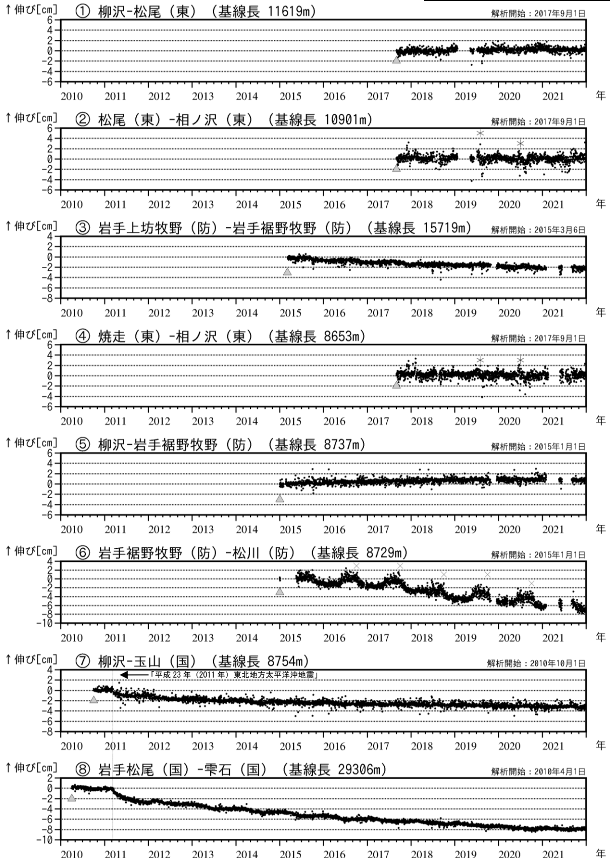
図3 岩手山 GNSS 基線長変化図 (2010年4月～2021年12月)
