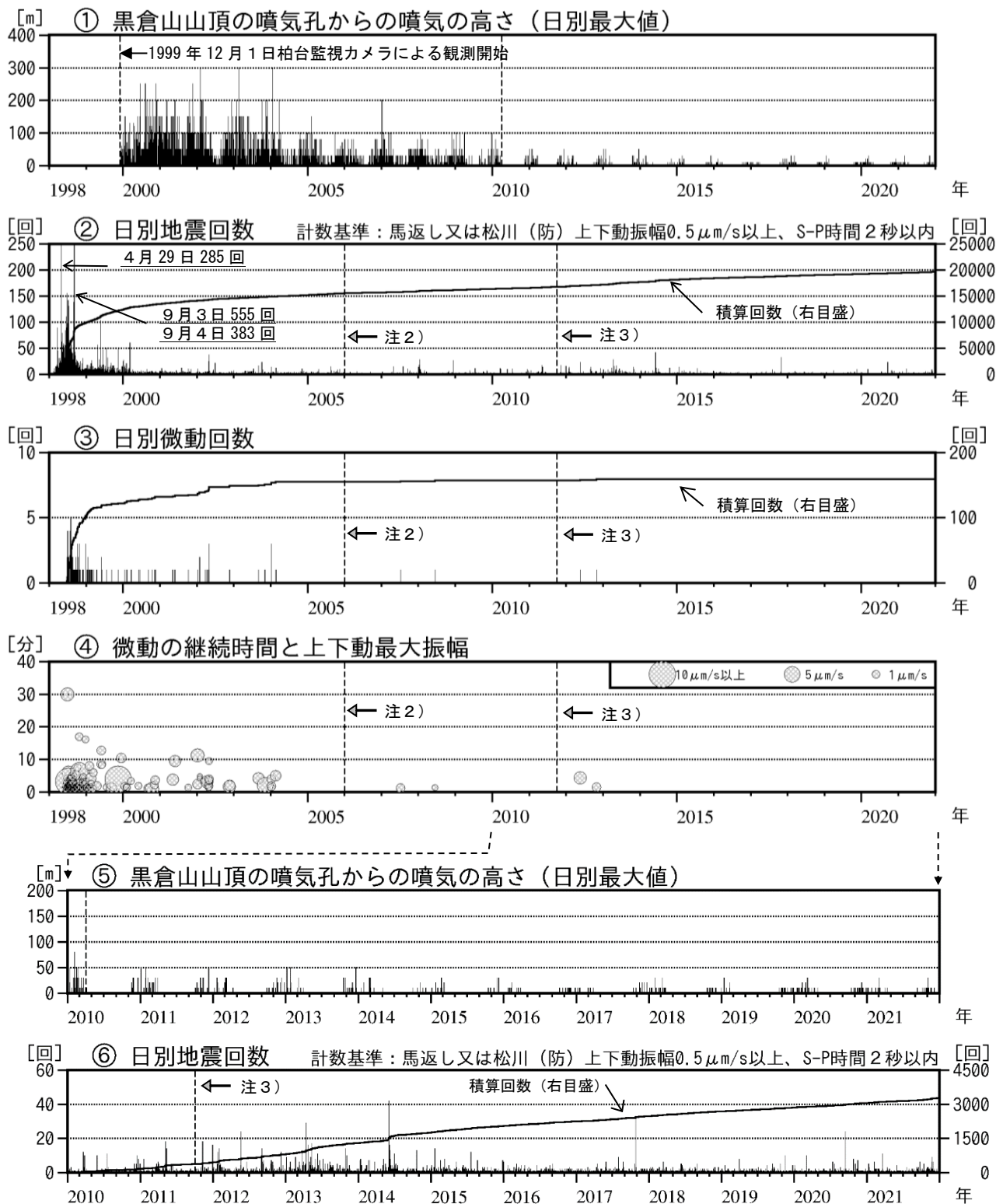
図2 岩手山 火山活動経過図（1998年1月～2021年12月）
