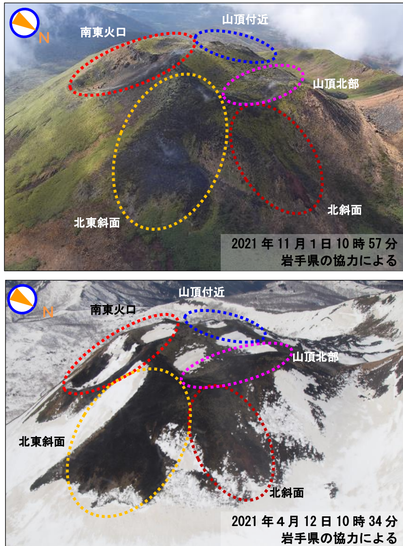
図4 秋田駒ヶ岳 上空からの女岳南東火口、北東斜面、北斜面、山頂北部及び山頂付近の状況 ・図中の破線の色は、図2の線の色に対応します。
