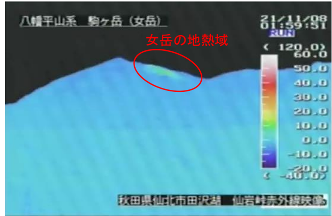
図1 秋田駒ヶ岳 女岳周辺の噴気と地表面温度分布の状況（可視：11月6日、赤外：11月8日） ・東北地方整備局が設置している仙岩峠監視カメラ（女岳山頂の南約5km）の可視及び赤外映像です。
