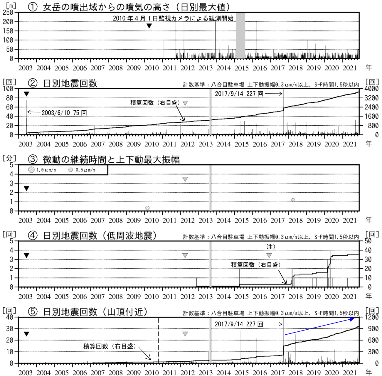
図5 秋田駒ヶ岳 火山活動経過図（2003年6月～2021年11月）
