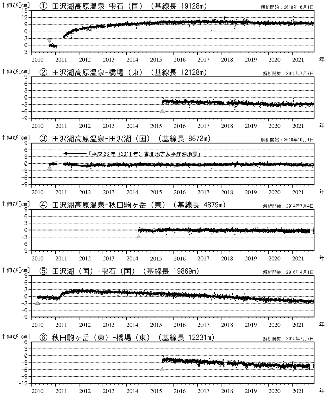
図8 秋田駒ヶ岳 GNSS 基線長変化図（2010年4月～2021年11月）
