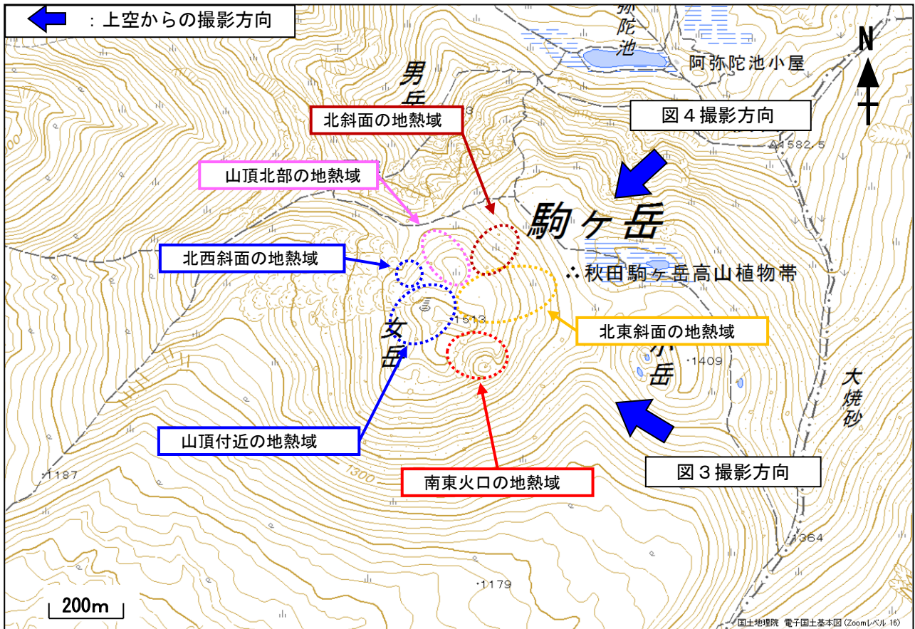
図2 秋田駒ヶ岳 女岳の地熱域の分布及び上空からの写真の撮影方向
