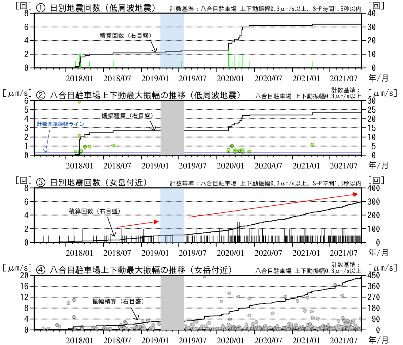
図6 秋田駒ヶ岳 低周波地震及び女岳付近の日別回数と最大振幅（2017年8月～2021年11月）
