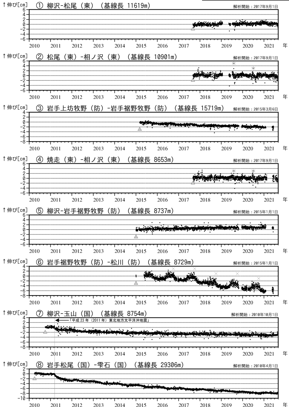
図4 岩手山 GNSS 基線長変化図 (2010年4月～2021年8月)
