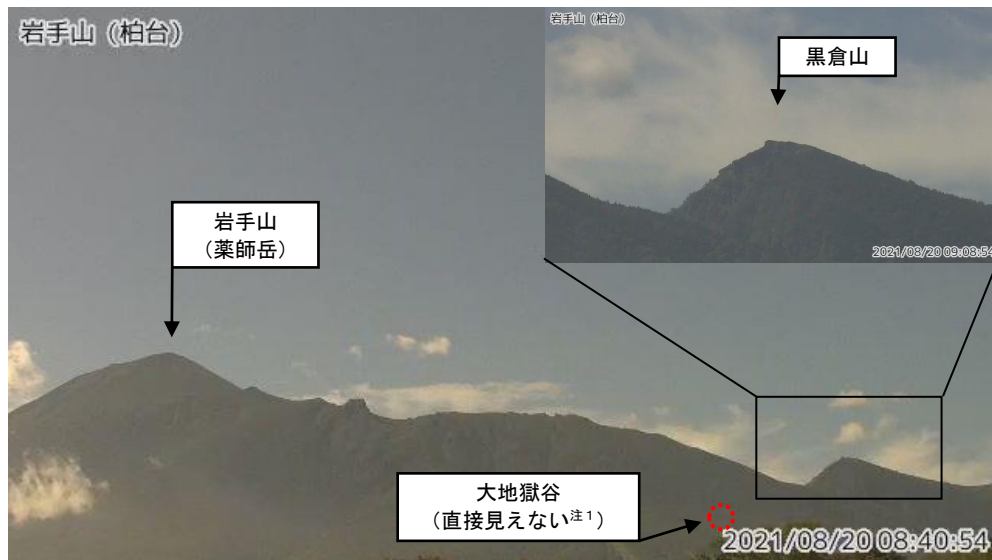
図1 岩手山 山頂部から黒倉山周辺の状況（8月20日）
