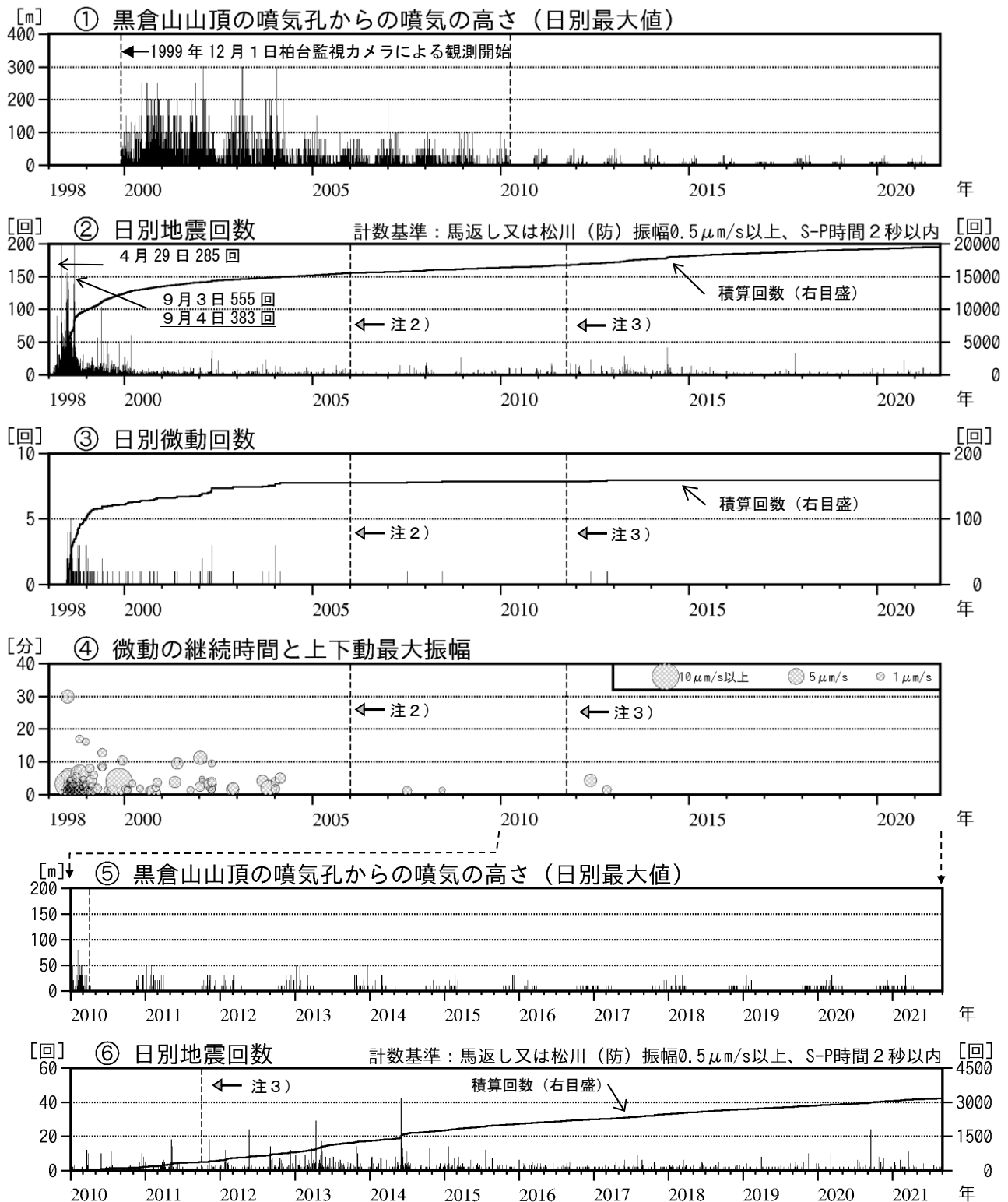
図3 岩手山 火山活動経過図（1998年1月～2021年8月）
