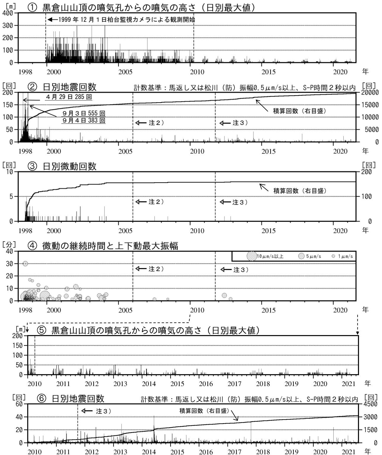
図3 岩手山 火山活動経過図（1998年1月～2021年7月）
