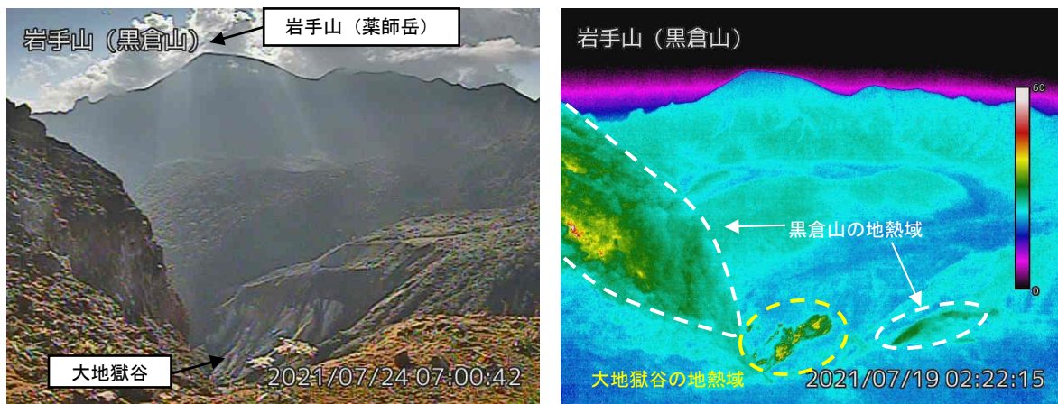
図2 岩手山 黒倉山監視カメラからの状況（7月24日）と地表面温度分布（7月19日）
