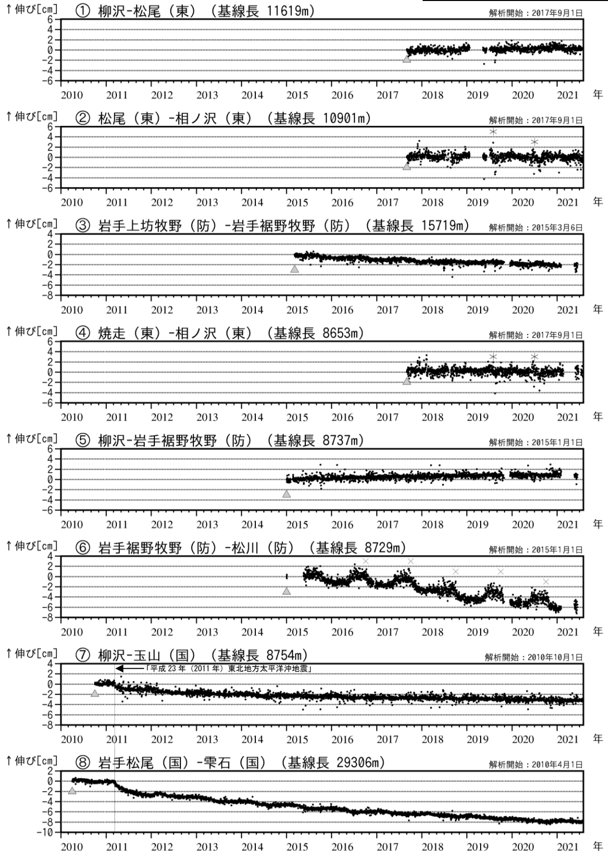
図4 岩手山 GNSS 基線長変化図 (2010年4月～2021年7月)
