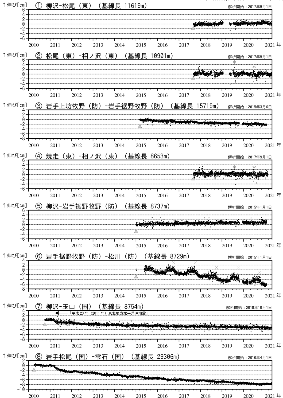
図7 岩手山 GNSS 基線長変化図 (2010年4月~2021年4月)
