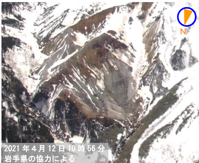
図4 岩手山 上空からの大地獄谷の状況
