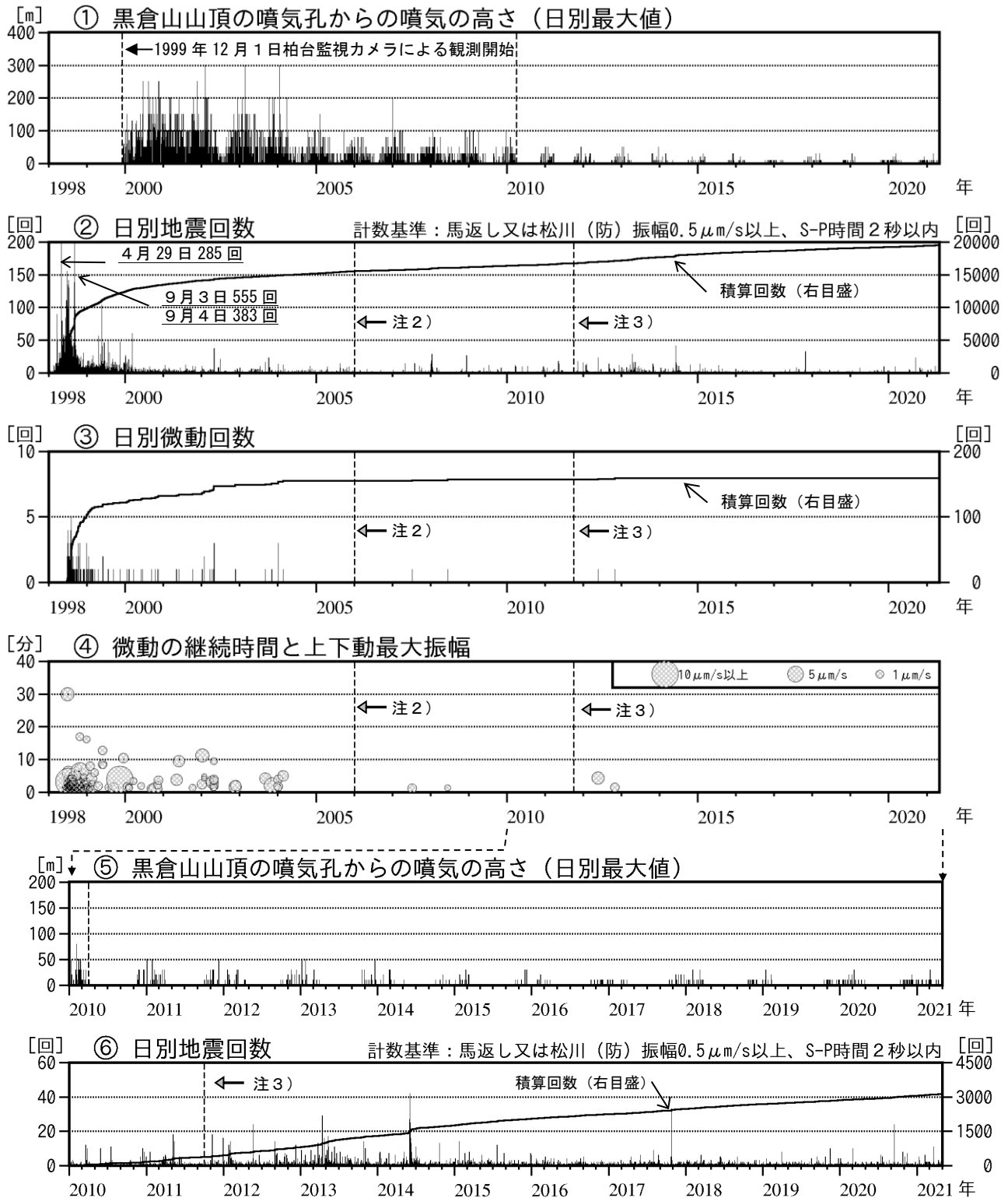
図6 岩手山 火山活動経過図（1998年1月～2021年4月）
