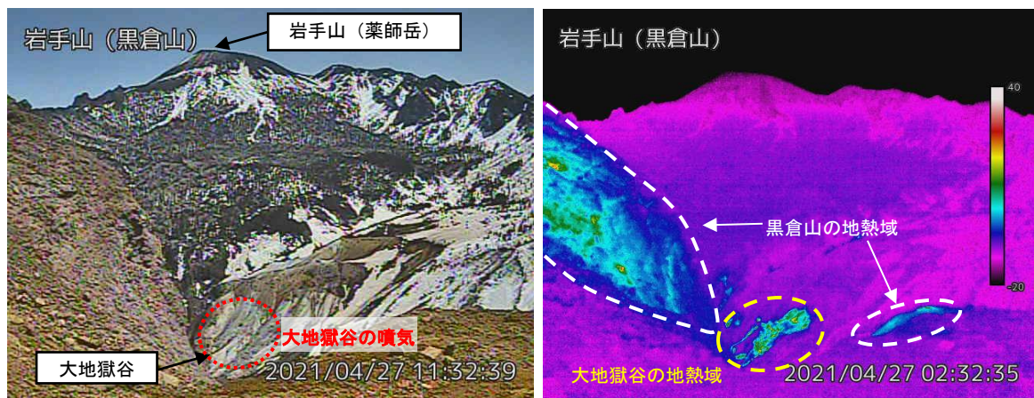
図2 岩手山 黒倉山監視カメラからの状況と地表面温度分布（4月27日）
