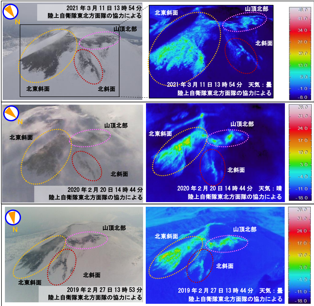
図3 秋田駒ヶ岳 上空からの女岳山頂北部、北東斜面及び北斜面の状況と地表面温度分布
