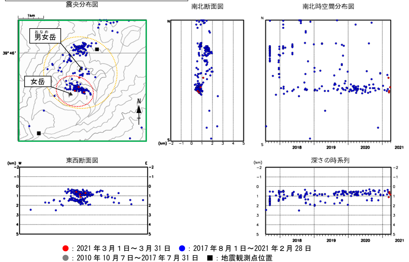
図7 秋田駒ヶ岳 地震活動（2010年10月7日～2021年3月）
