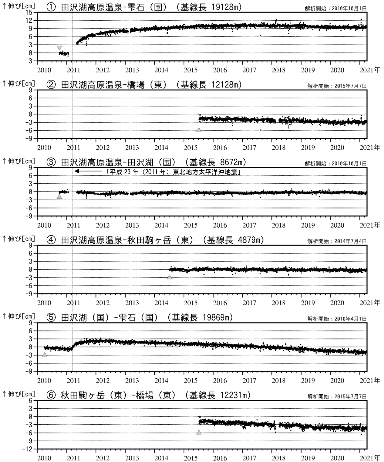
図8 秋田駒ヶ岳 GNSS 基線長変化図 (2010年4月～2021年3月)
