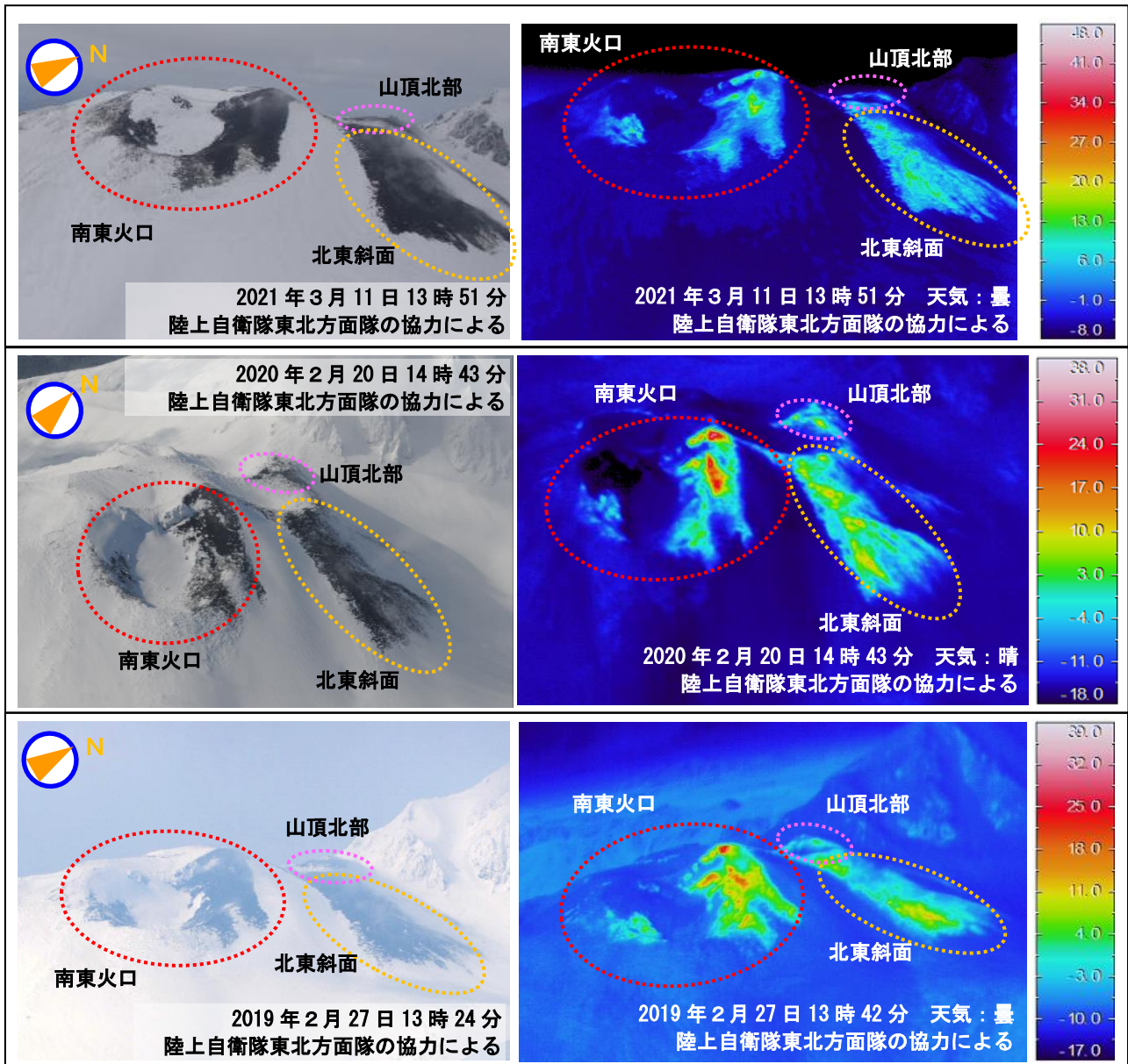
図4 秋田駒ヶ岳 上空からの南東火口の状況と地表面温度分布
