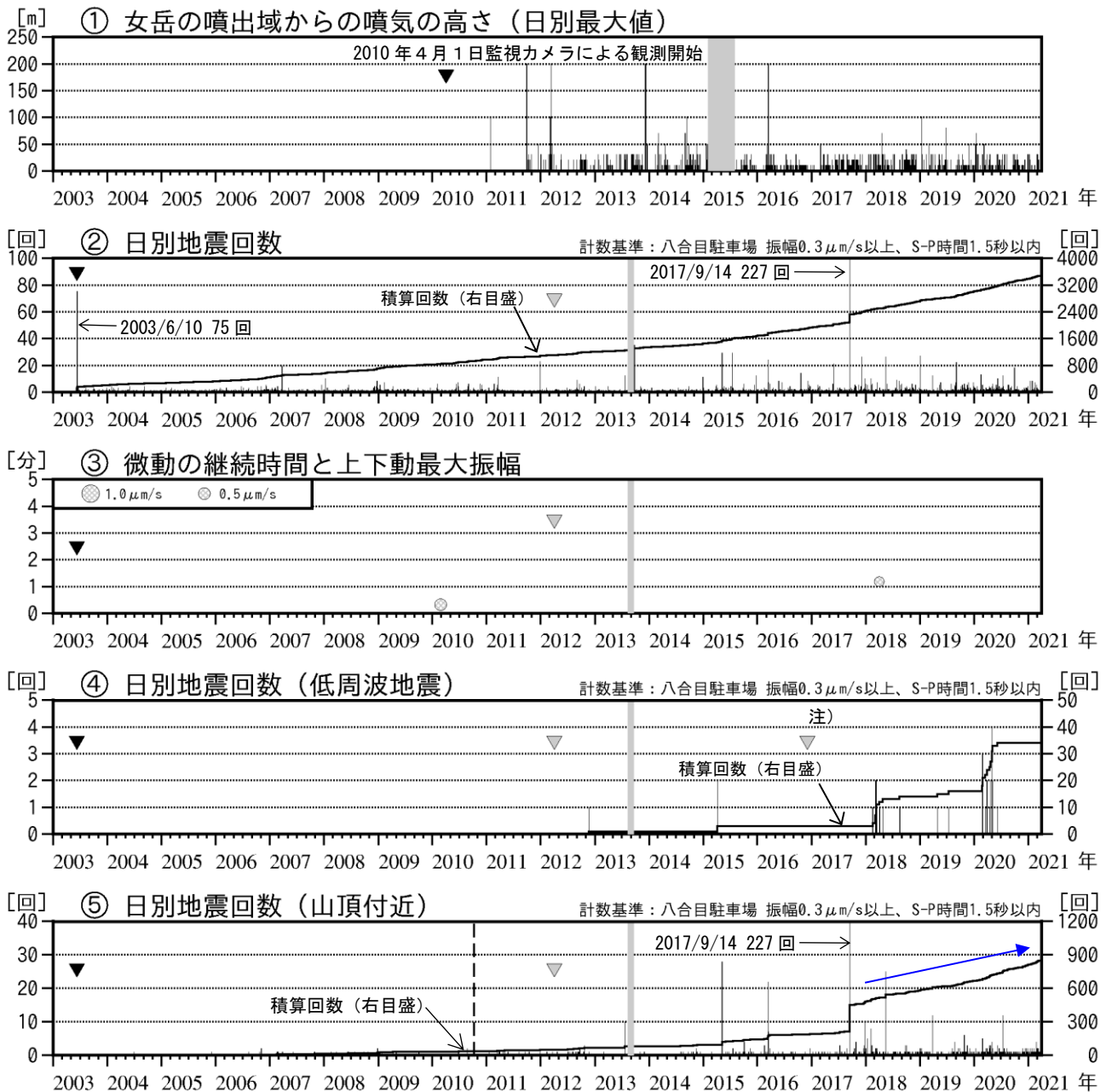
図5 秋田駒ヶ岳 火山活動経過図（2003年6月～2021年3月）
