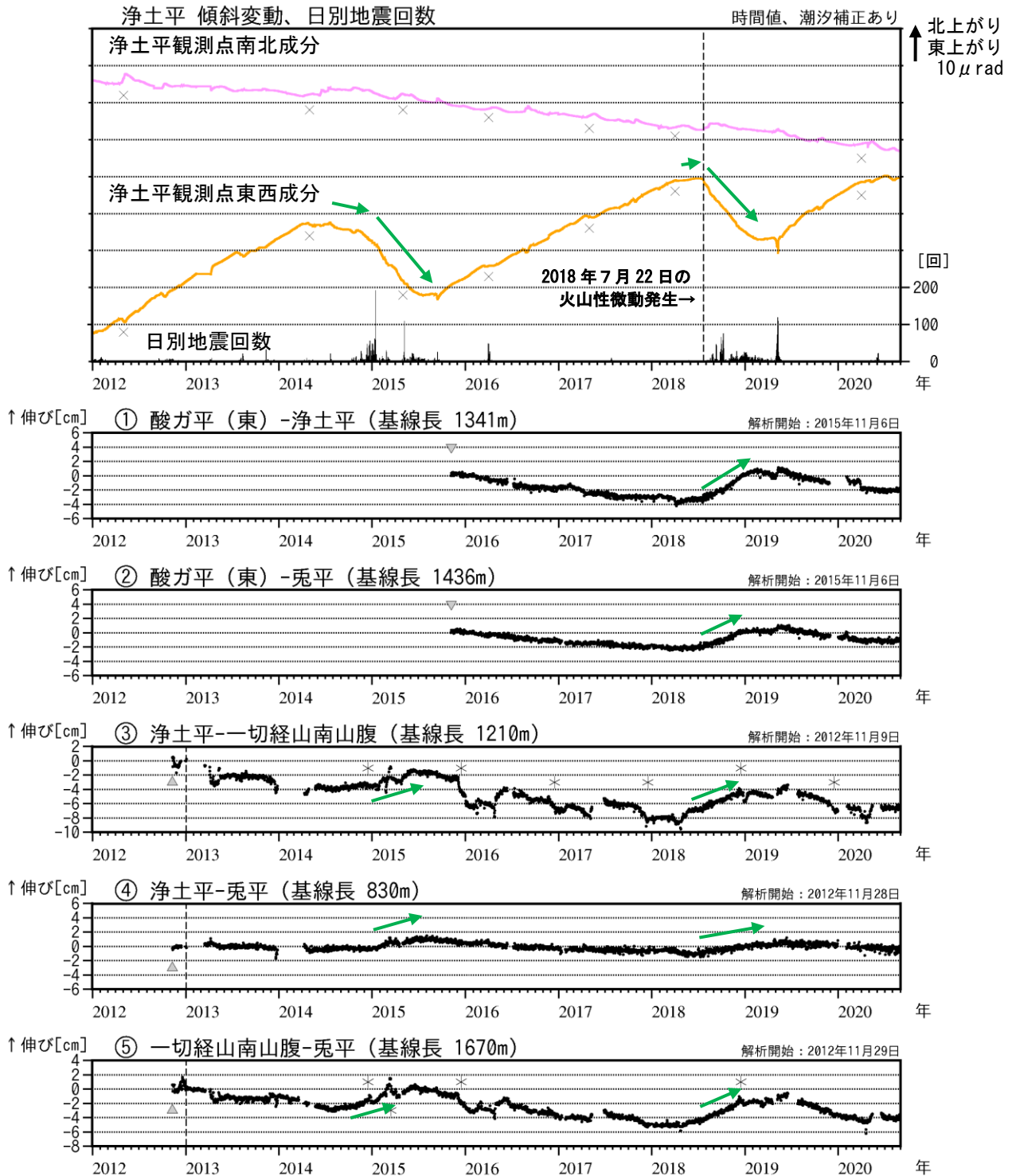
図6 吾妻山 大穴火口浅部の地殻変動(2012年1月~2020年8月)
