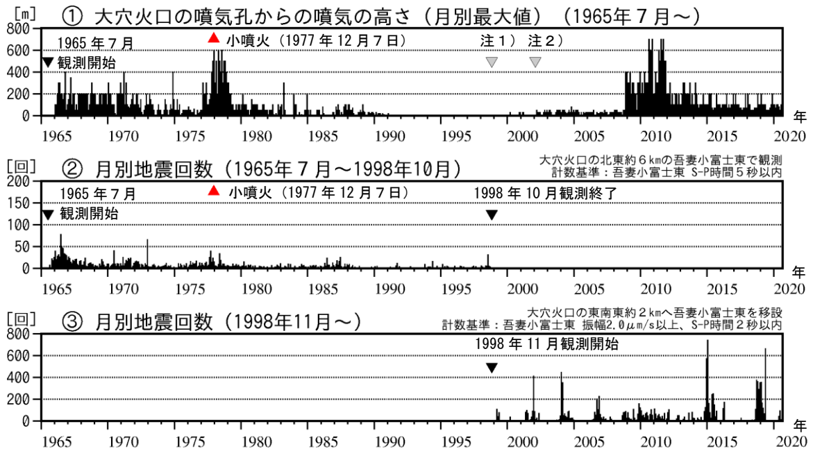
図1 吾妻山 長期的な火山活動の経過（1965年7月～2020年8月）
