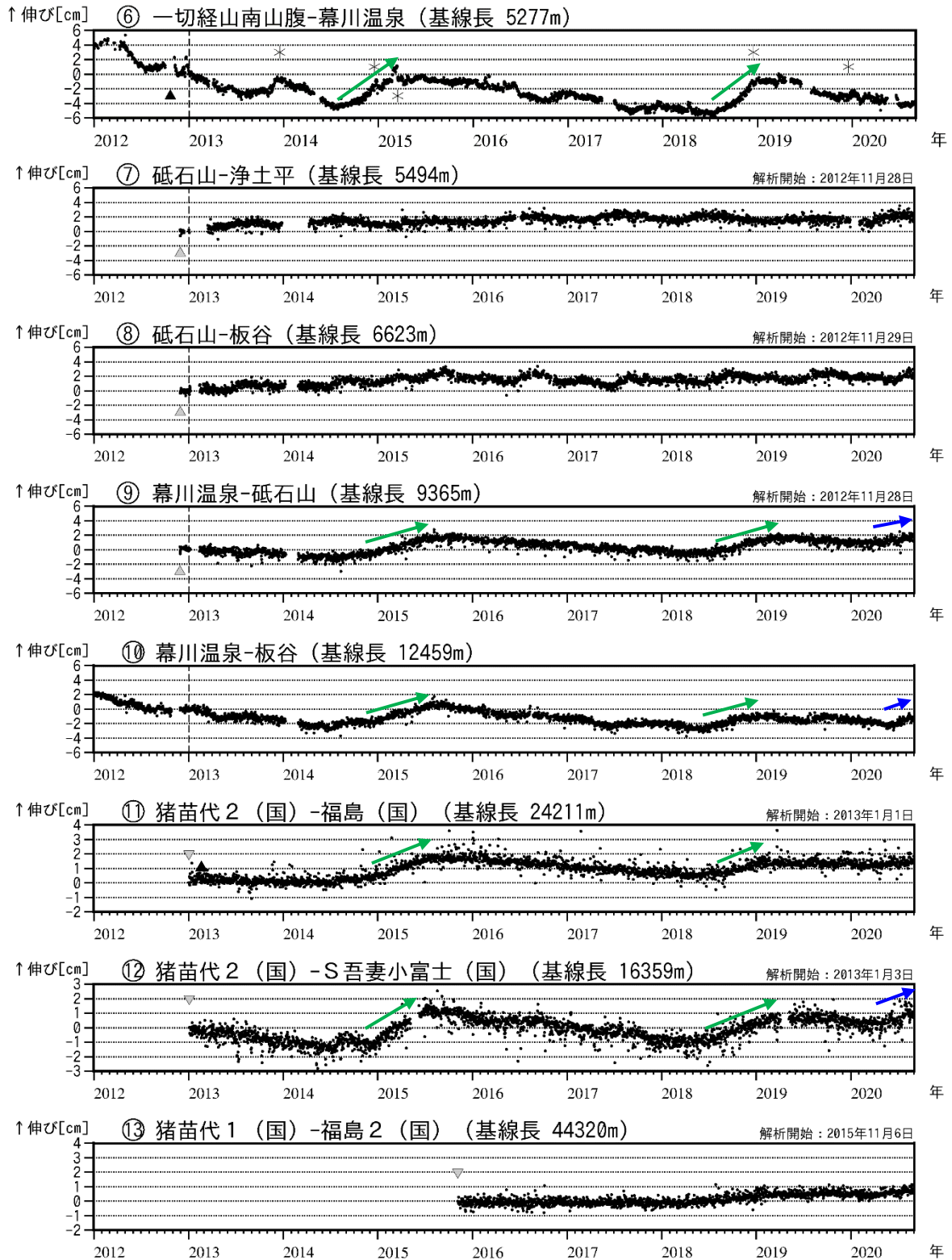
図7 吾妻山 吾妻山深部の地殻変動（2012年1月～2020年8月）
