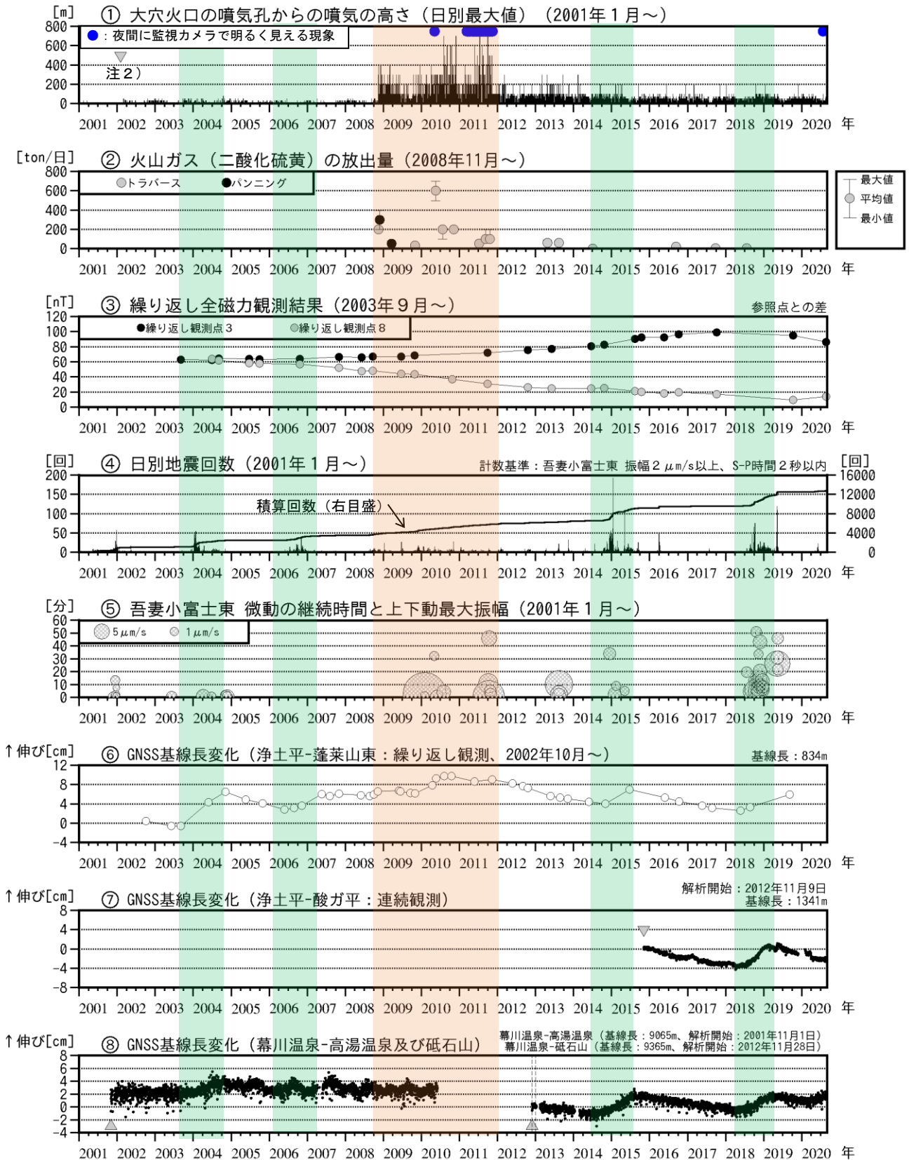
図2 吾妻山 中期的な火山活動の経過（2001年1月～2020年8月）
