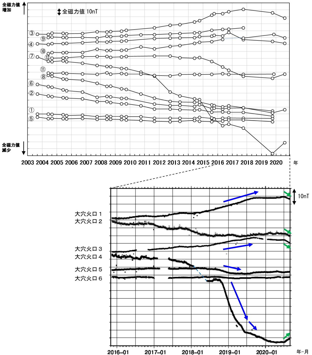
図 15 吾妻山 全磁力繰り返し観測（上）及び連続観測（下）の全磁力値変化 （2003年9月～2020年8月）
