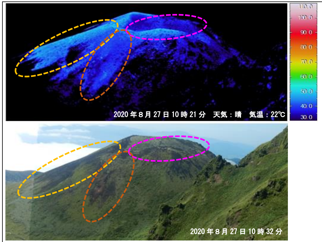
図3 秋田駒ヶ岳 北方向から撮影した女岳の状況と地表面温度分布
