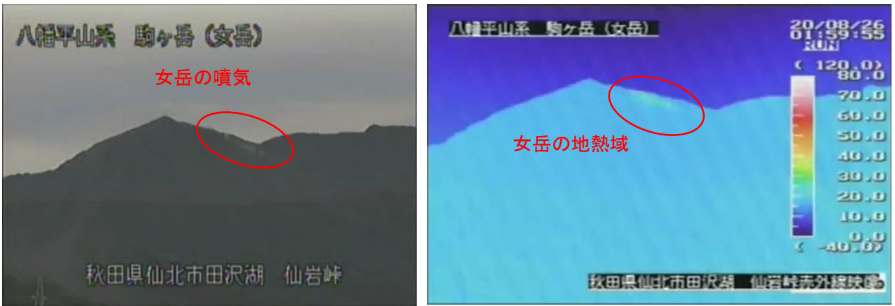
図1 秋田駒ヶ岳 女岳周辺の噴気と地表面温度分布の状況（可視：8月8日、赤外：8月26日） ※東北地方整備局が設置している仙岩峠監視カメラ（女岳山頂の南約5km）の可視及び赤外映像です。
