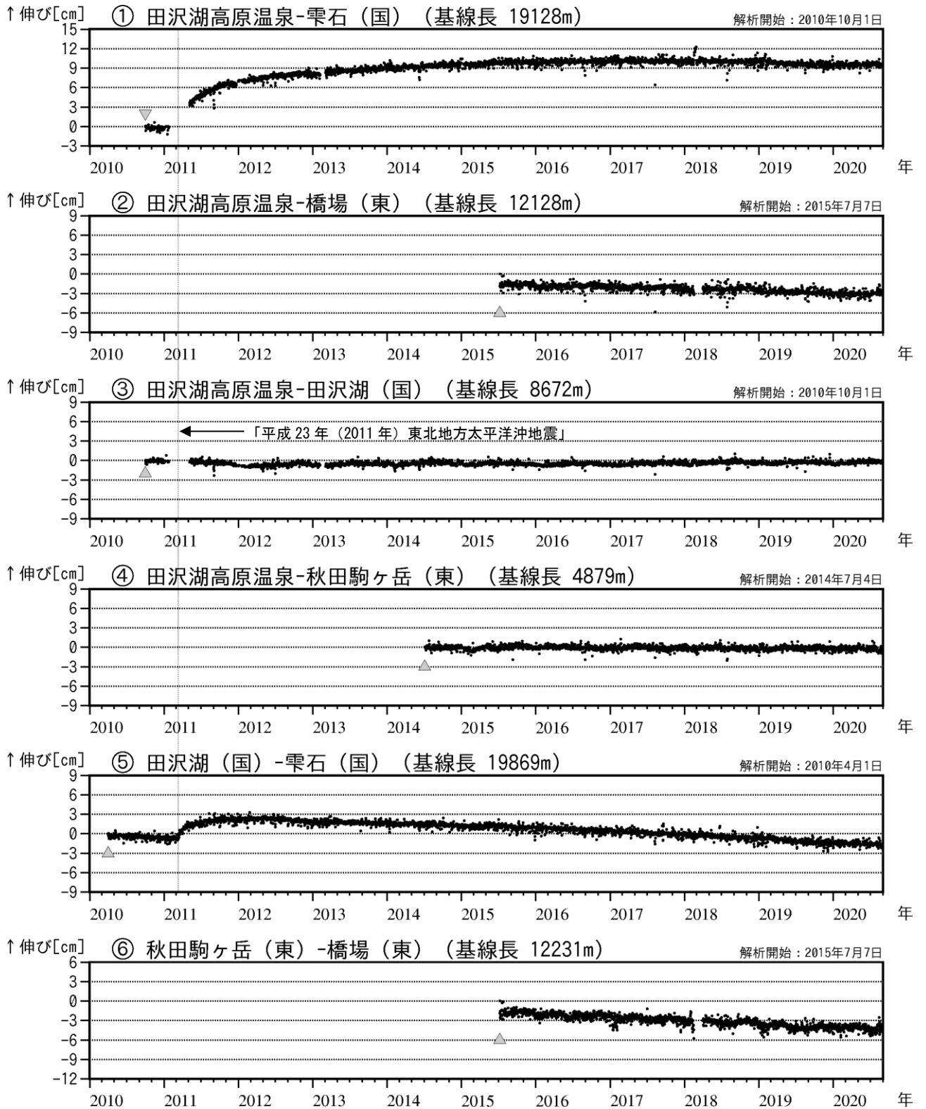
図9 秋田駒ヶ岳 GNSS 基線長変化図 (2010年4月～2020年8月)
