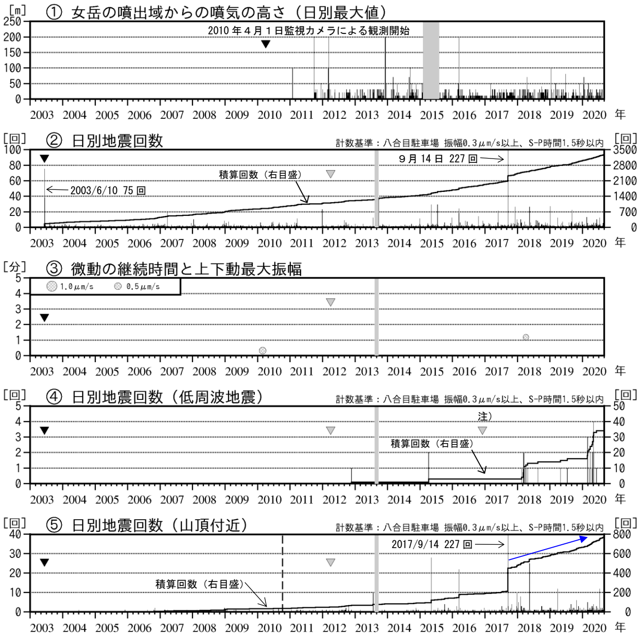
図6 秋田駒ヶ岳 火山活動経過図（2003年6月～2020年8月）
