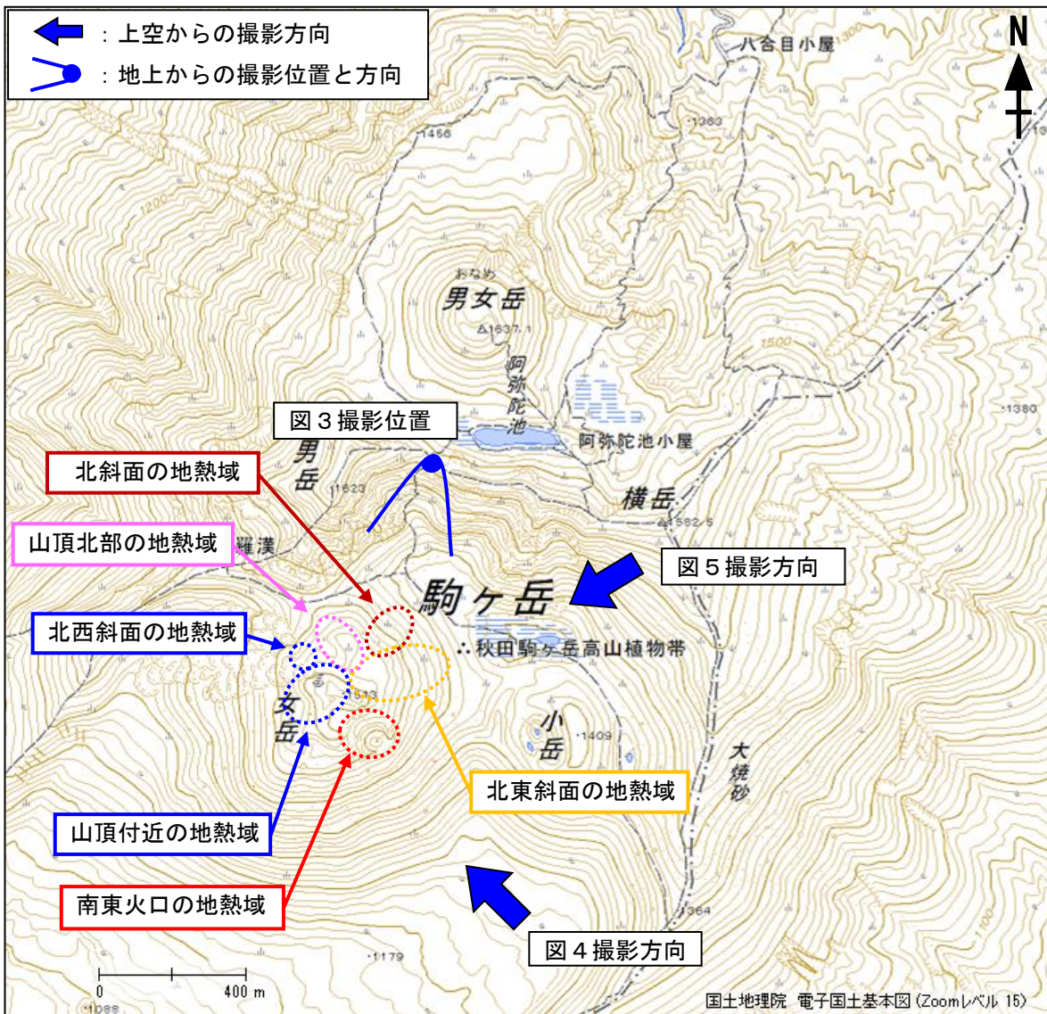
図2 秋田駒ヶ岳 女岳の地熱域の分布及び写真と地表面温度分布撮影方向
