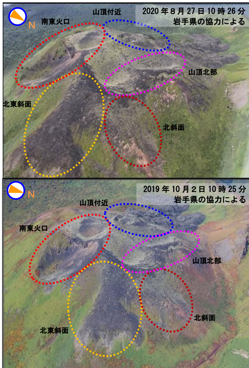
図5 秋田駒ヶ岳 上空から撮影した女岳南東火口、北東斜面、北斜面、山頂北部及び山頂付近の状況
