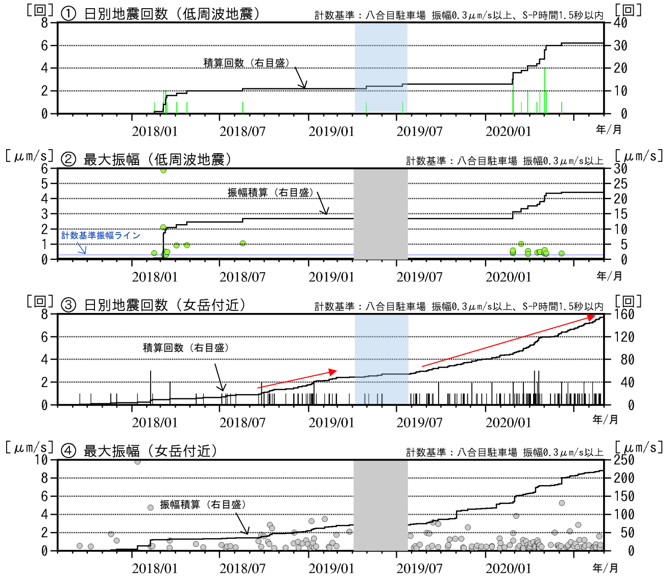
図7 秋田駒ヶ岳 低周波地震及び女岳付近の日別回数と最大振幅（2017年8月～2020年8月）
