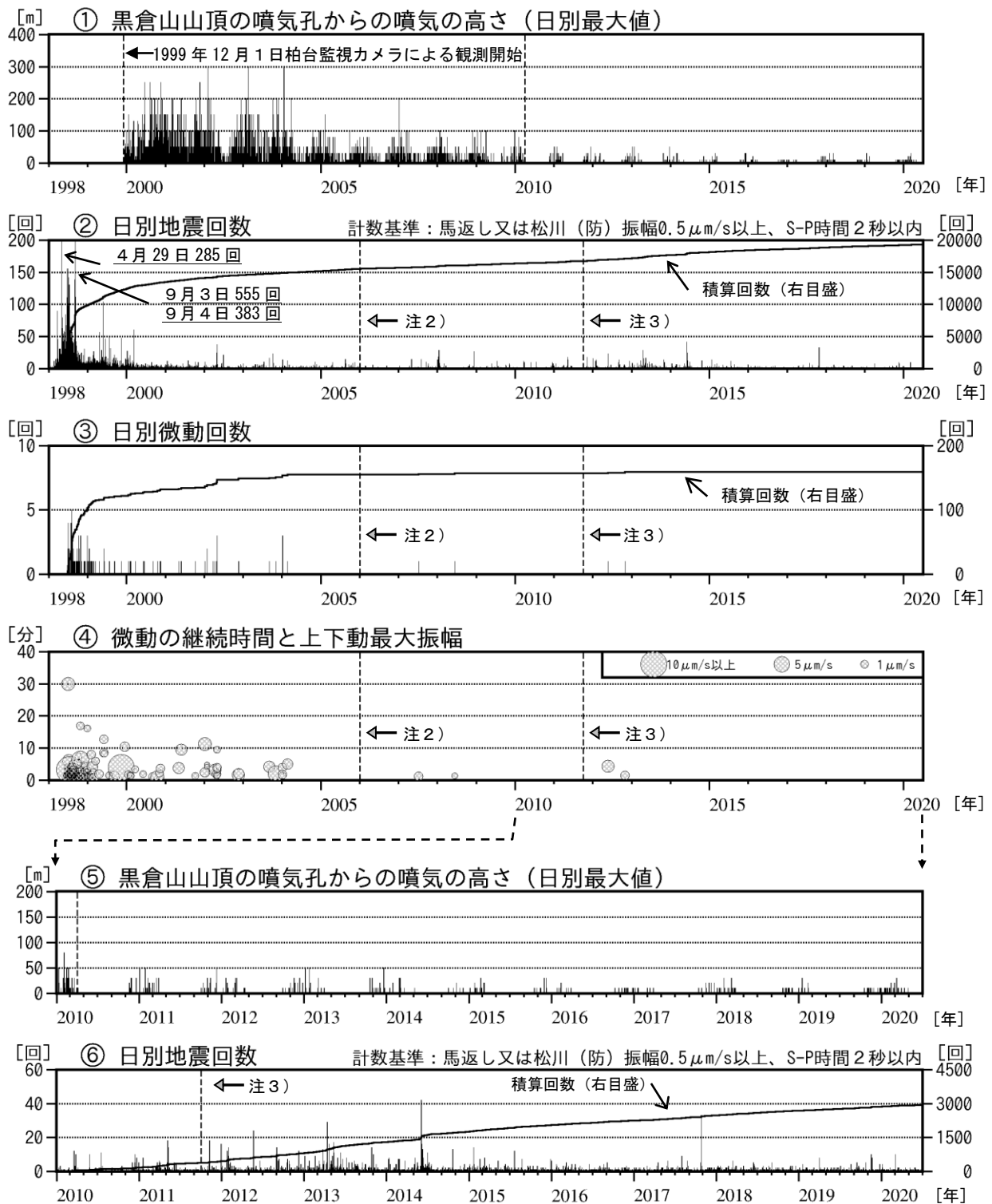
図3 岩手山 火山活動経過図（1998年1月～2020年6月）
