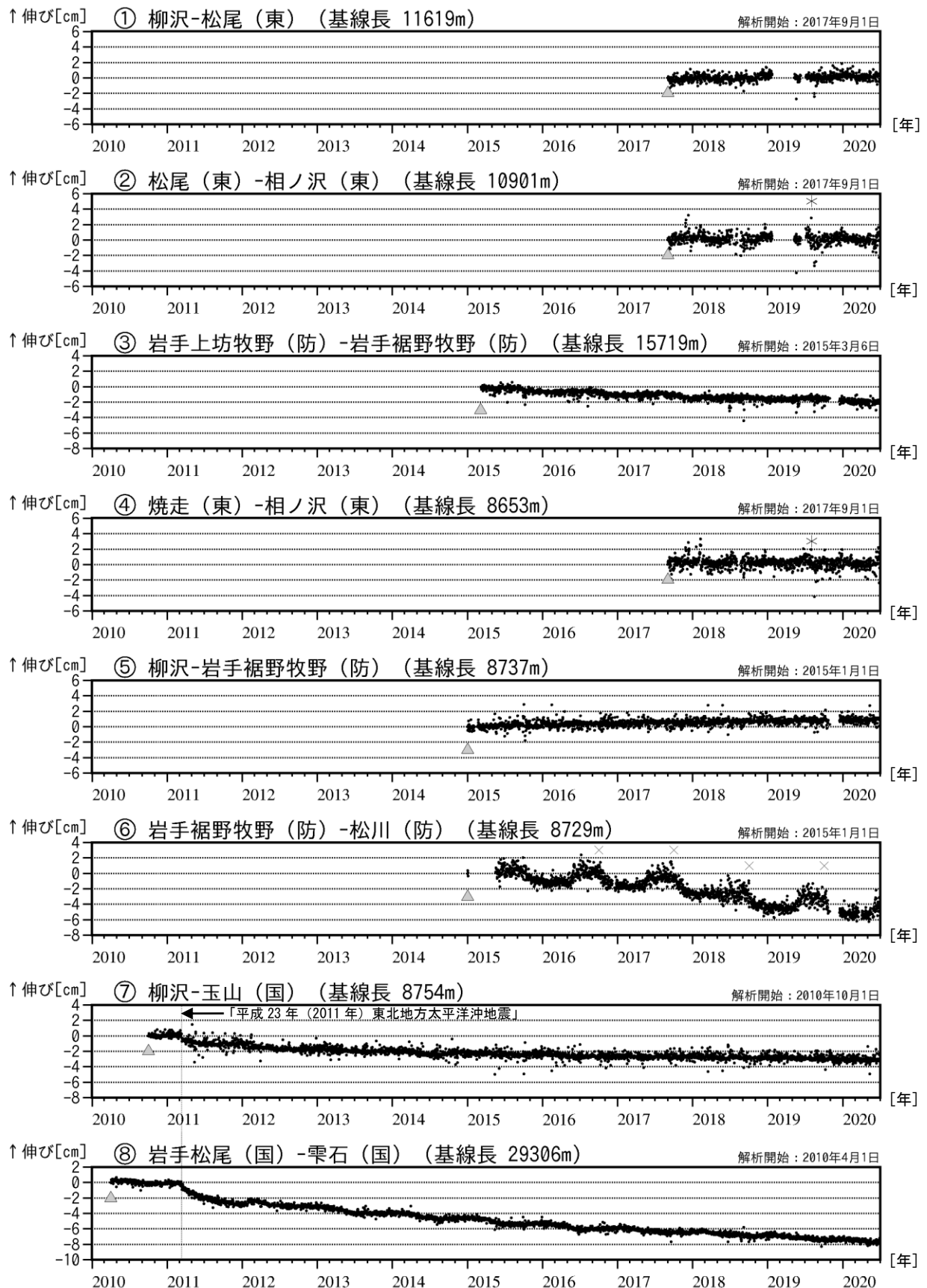
図4 岩手山 GNSS 基線長変化図 (2010年4月～2020年6月)
