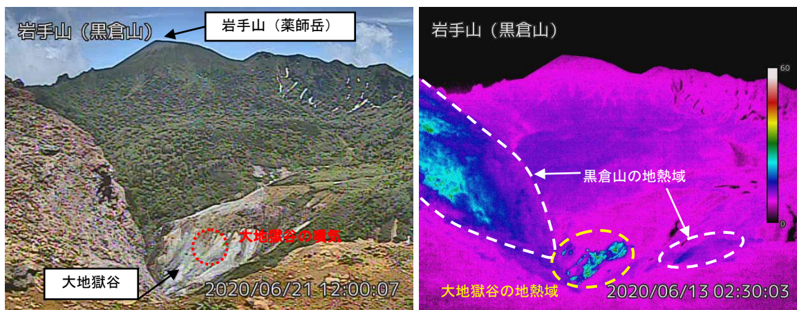
図2 岩手山 黒倉山監視カメラからの状況（6月21日）と地表面温度分布（6月13日）
