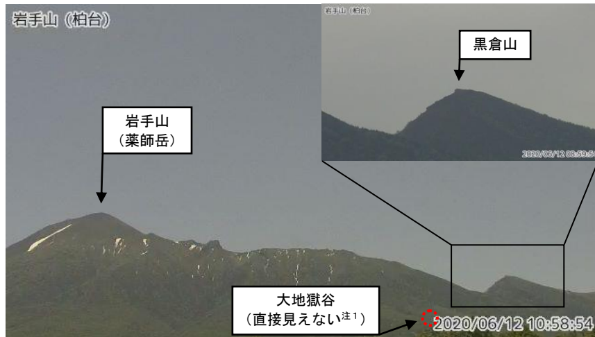
図1 岩手山 黒倉山の噴気の状況（6月12日）
