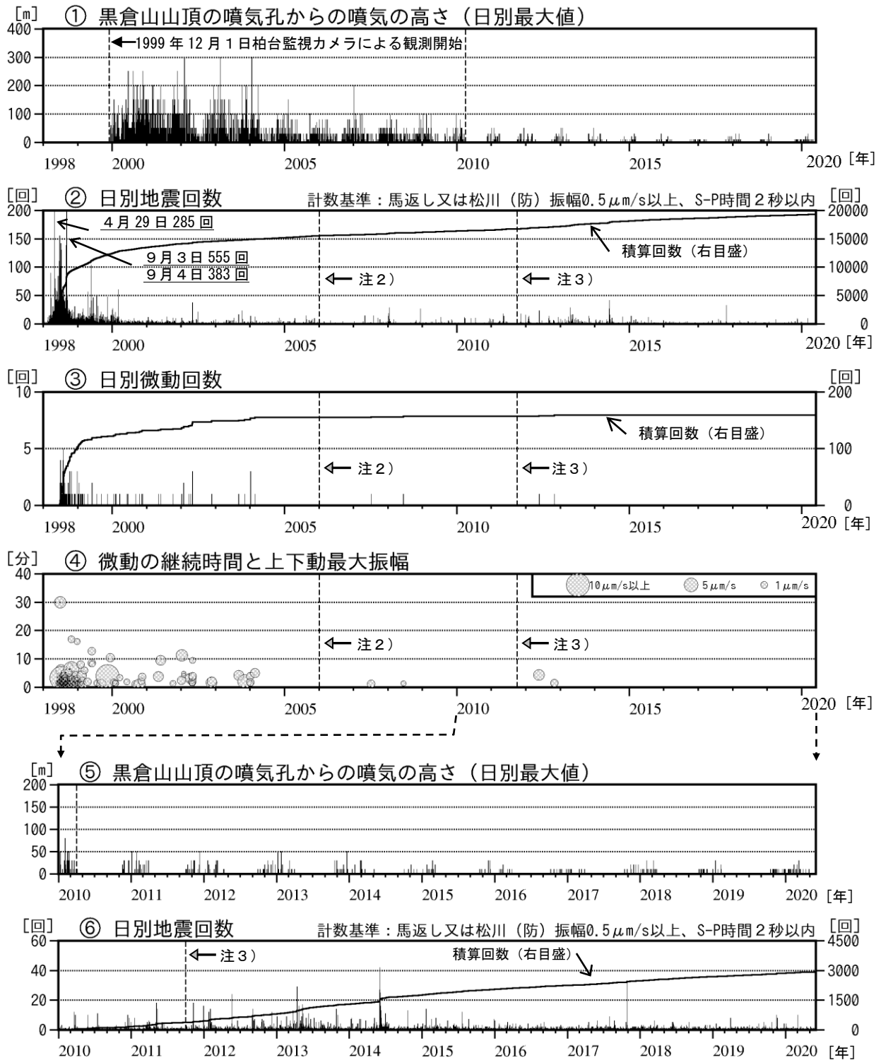
図3 岩手山 火山活動経過図（1998年1月～2020年5月）
