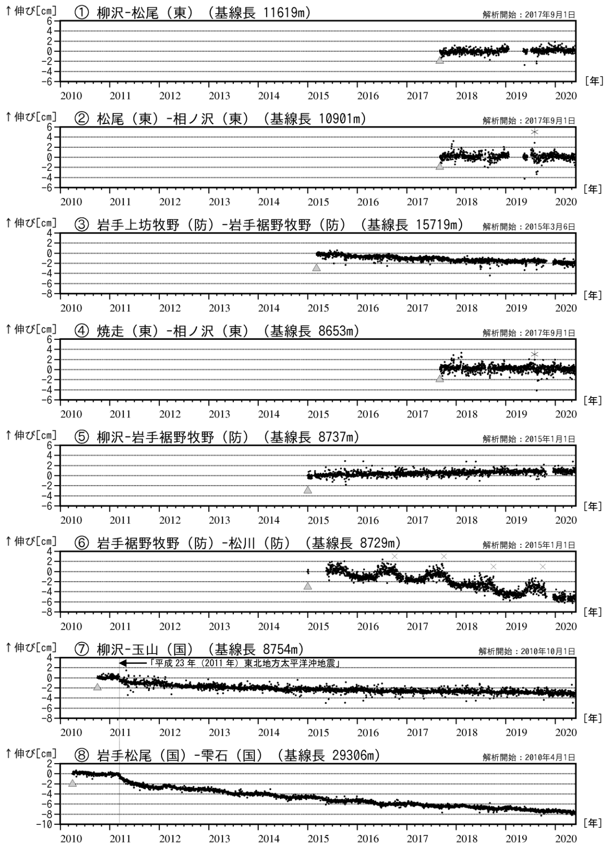
図4 岩手山 GNSS 基線長変化図 (2010年4月～2020年5月)
