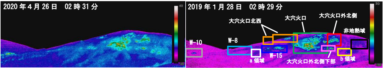
図5 吾妻山 浄土平3監視カメラ（熱映像）による大穴火口周辺の地熱域の状況
