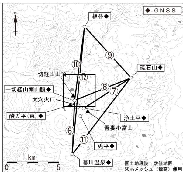
図4 吾妻山 GNSS 観測基線図
