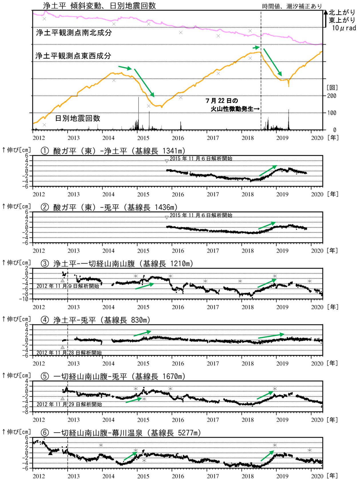
図2 吾妻山 傾斜変動及びGNSS基線長変化図（2012年1月～2020年4月）
