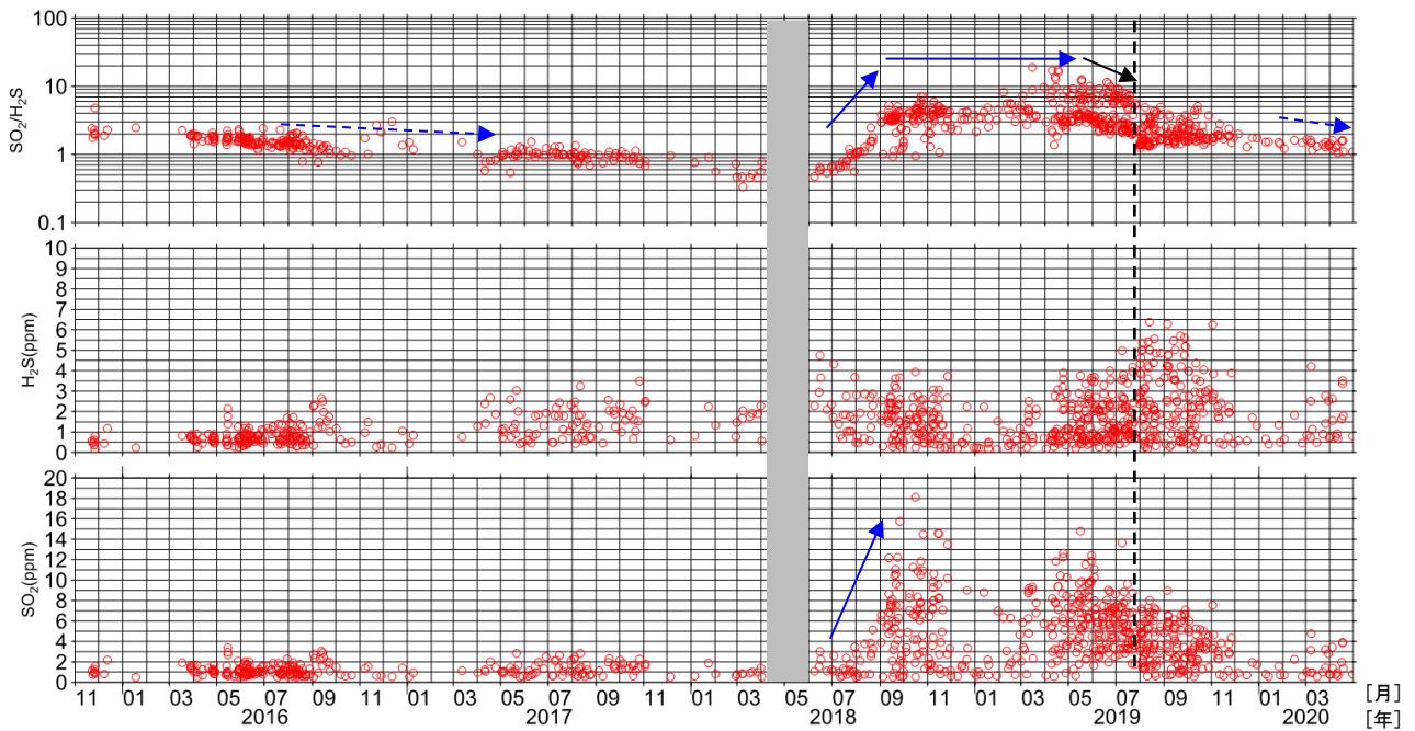
図8 吾妻山 火山ガス観測装置による観測（2015年11月～2020年4月）
