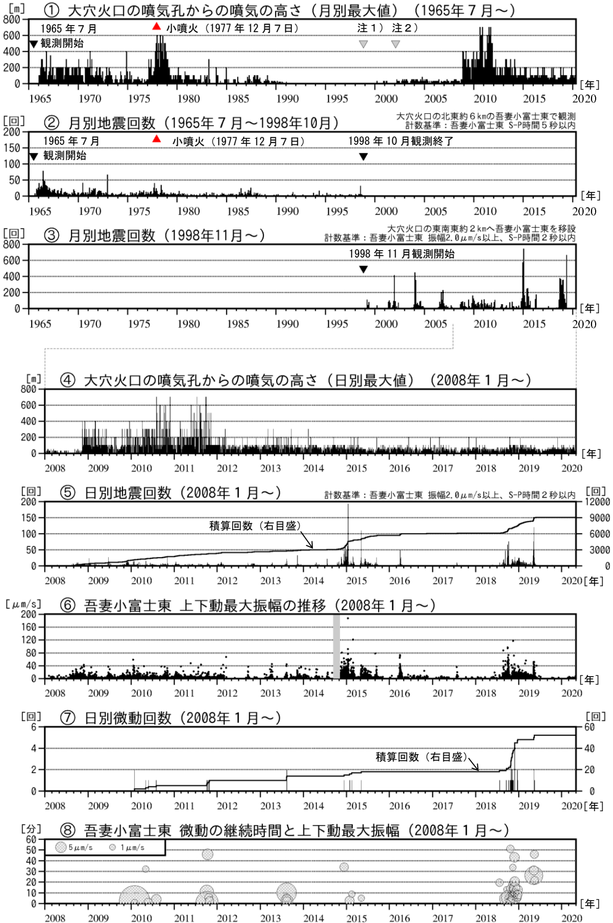
図1 吾妻山 火山活動経過図（1965年7月～2020年4月）
