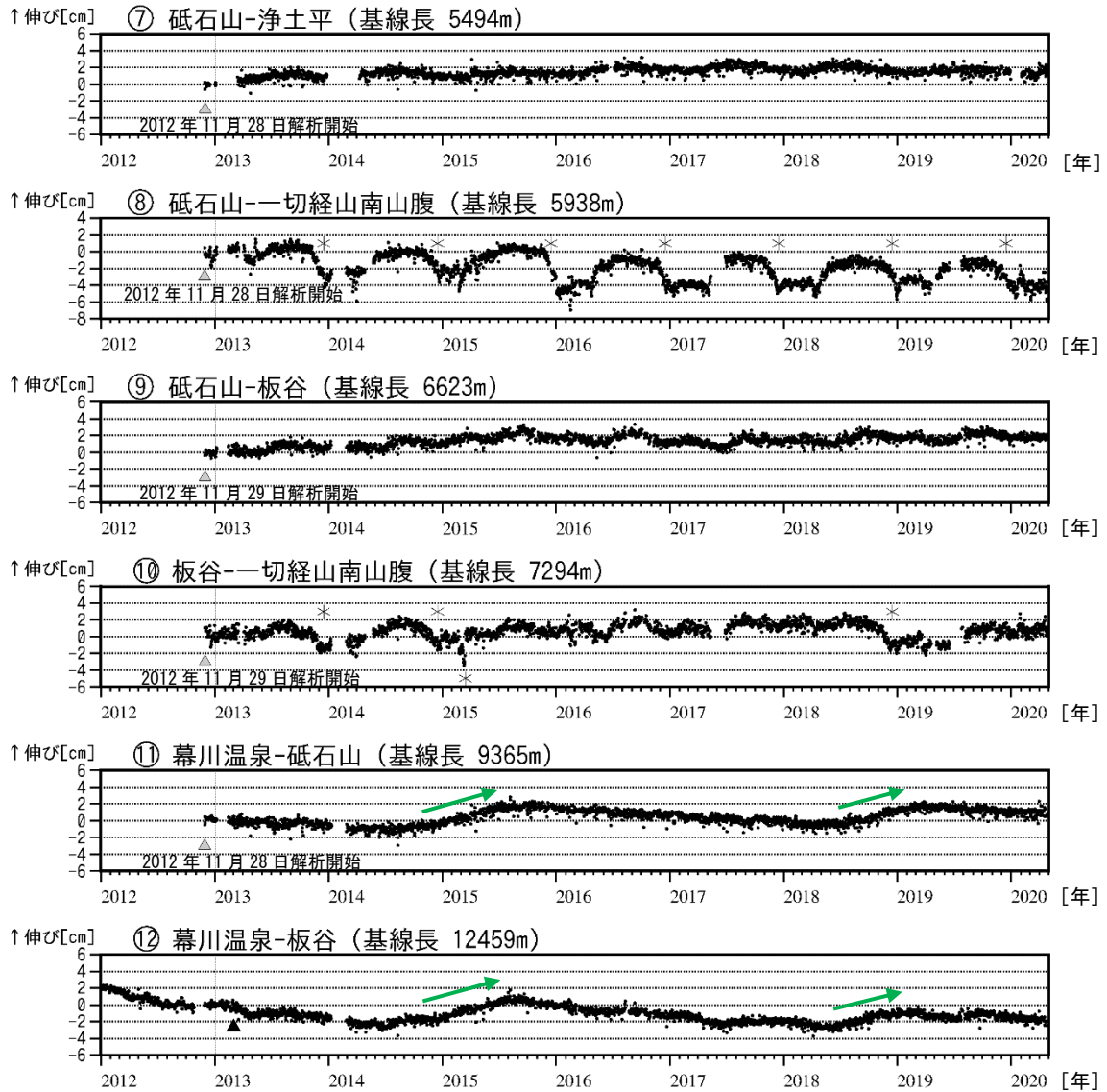
図3 吾妻山 GNSS 基線長変化図（2012年1月～2020年4月）
