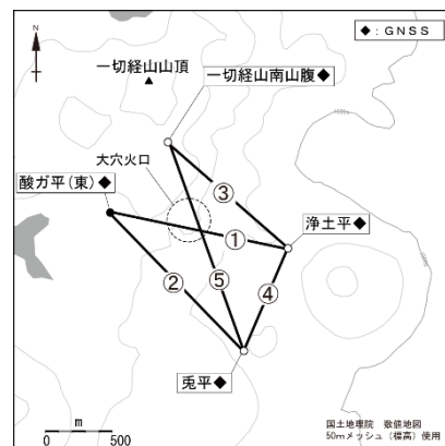
図4 吾妻山 GNSS 観測基線図
