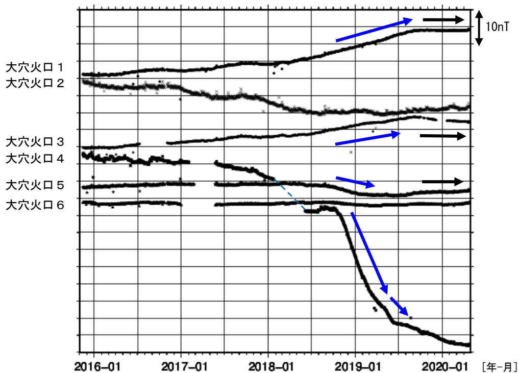
図10 吾妻山 全磁力連続観測点の全磁力値変化（2015年11月～2020年4月）
