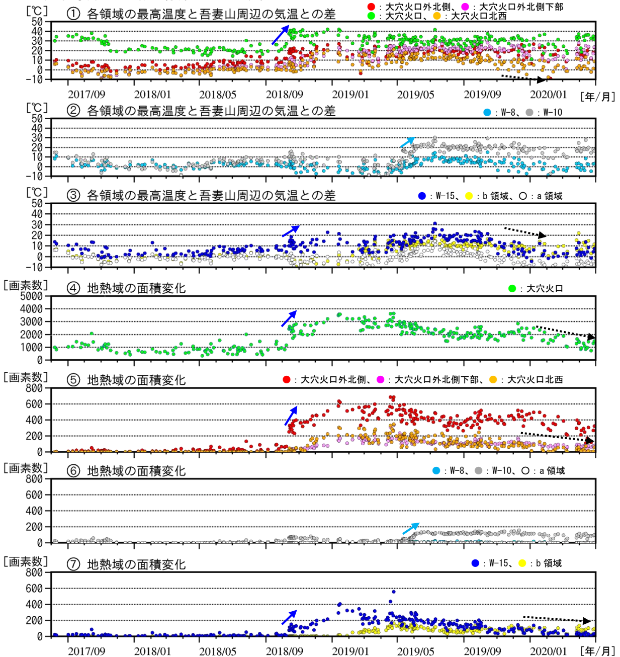
図6 吾妻山 監視カメラによる大穴火口周辺の地熱域の経過（2017年8月～2020年4月）
